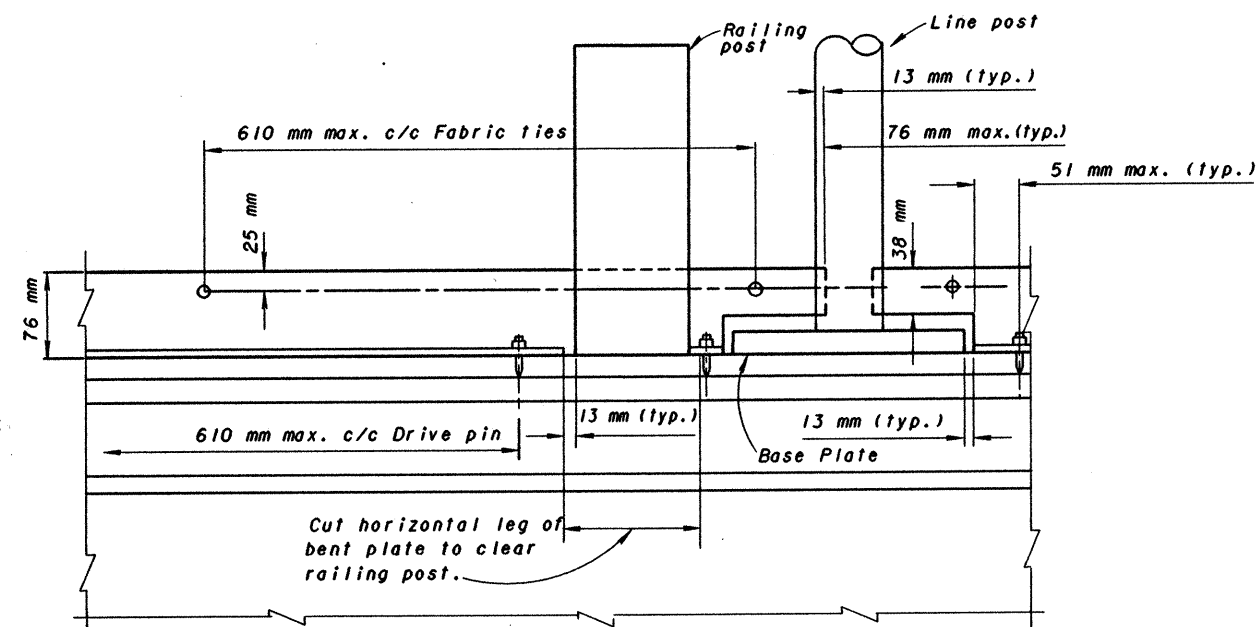
VIEW A-A
