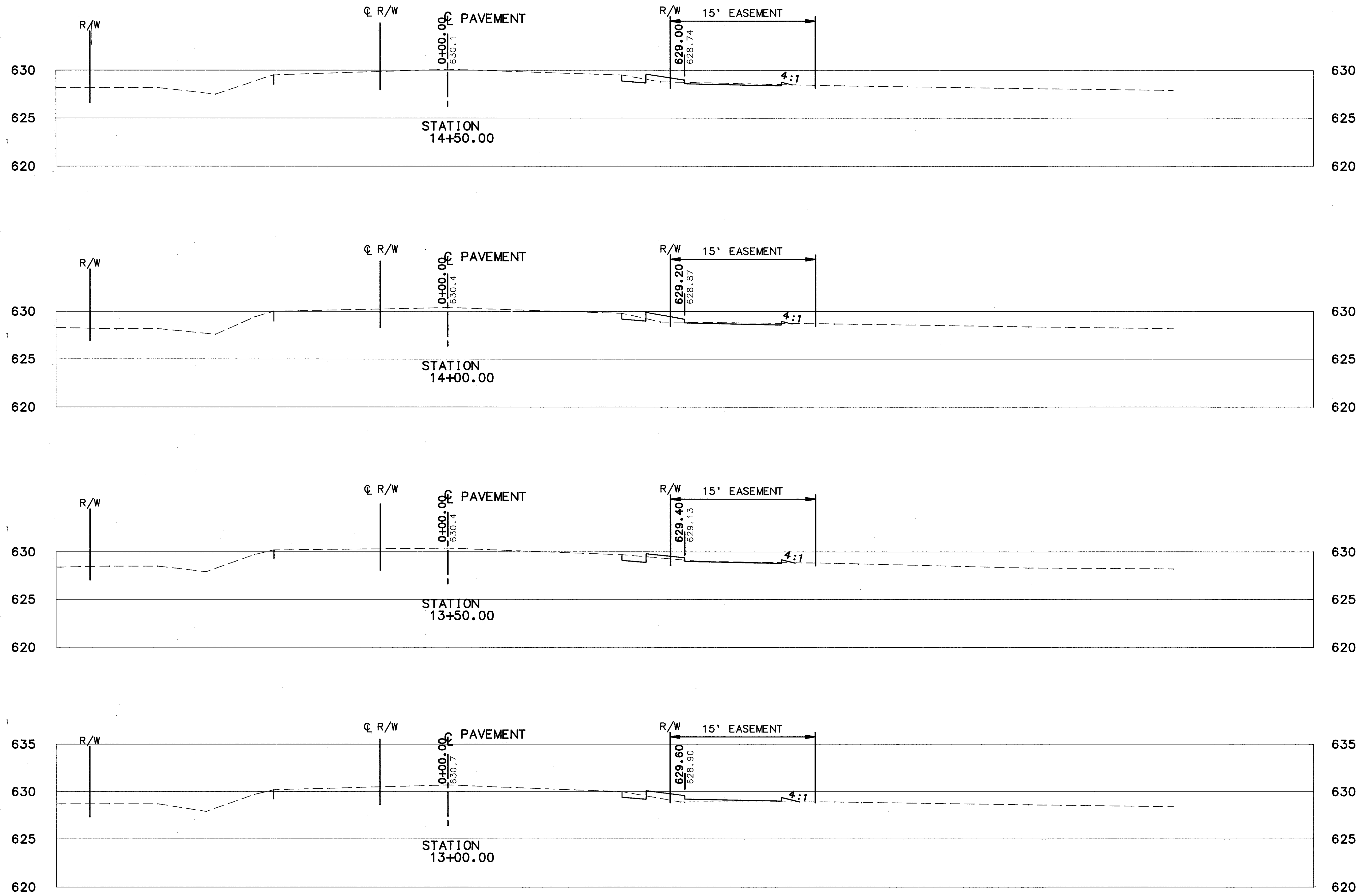
CROSS-SECTIONS STA. 13+00 TO STA. 14+50
