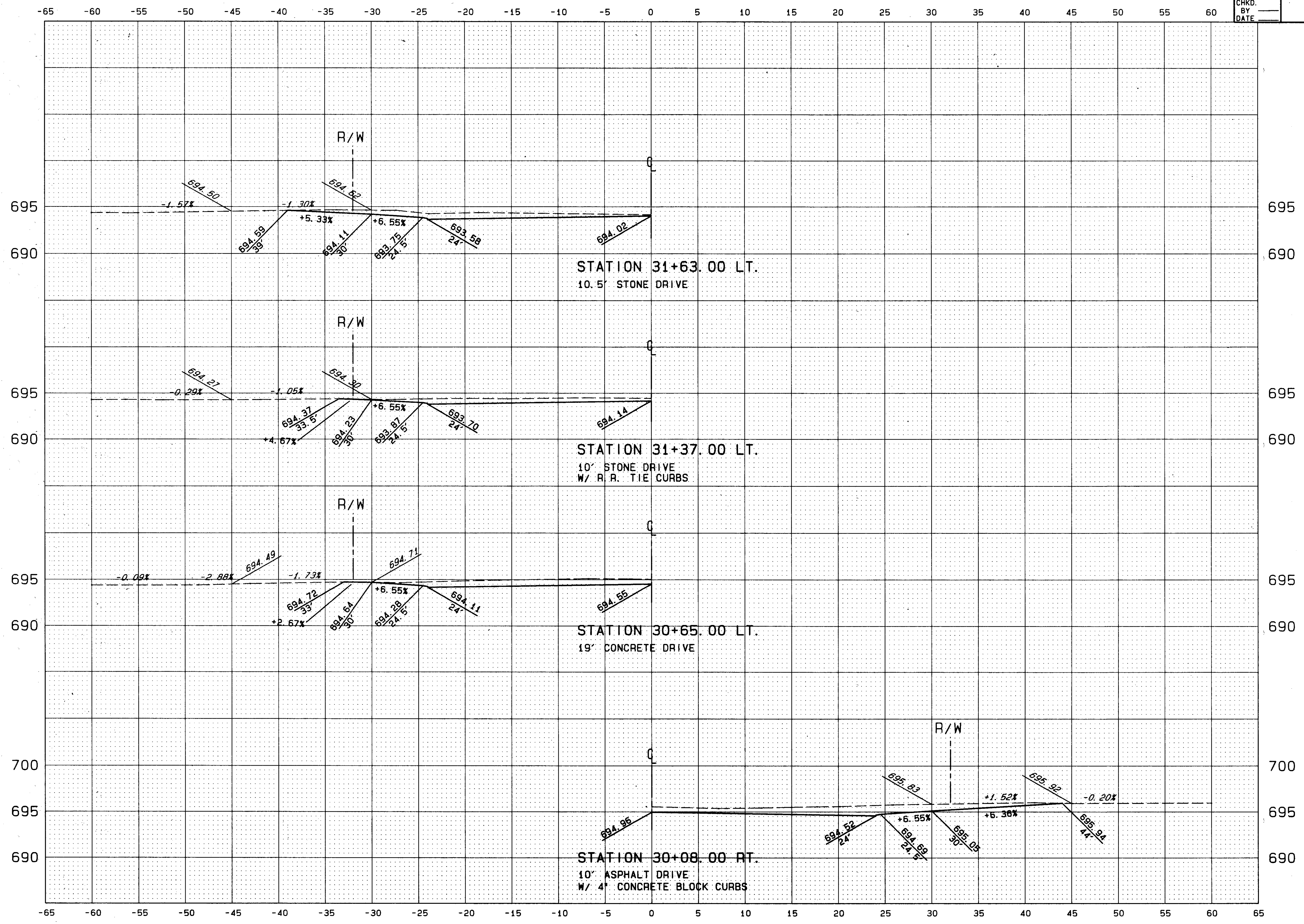
DRIVE PROFILES STA. 30+08 TO STA. 31+63
