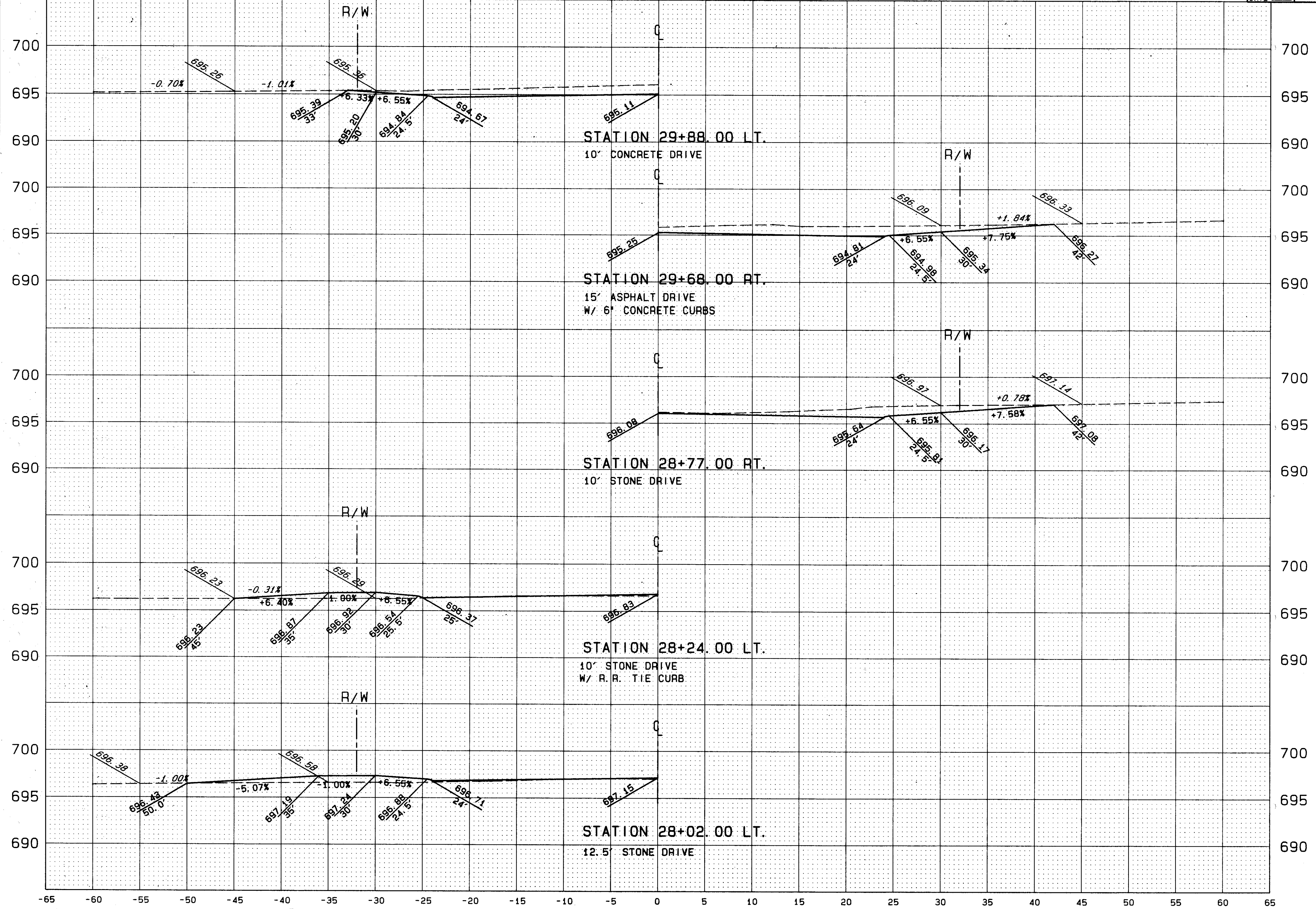
DRIVE PROFILES STA. 28+02 TO STA. 29+88
