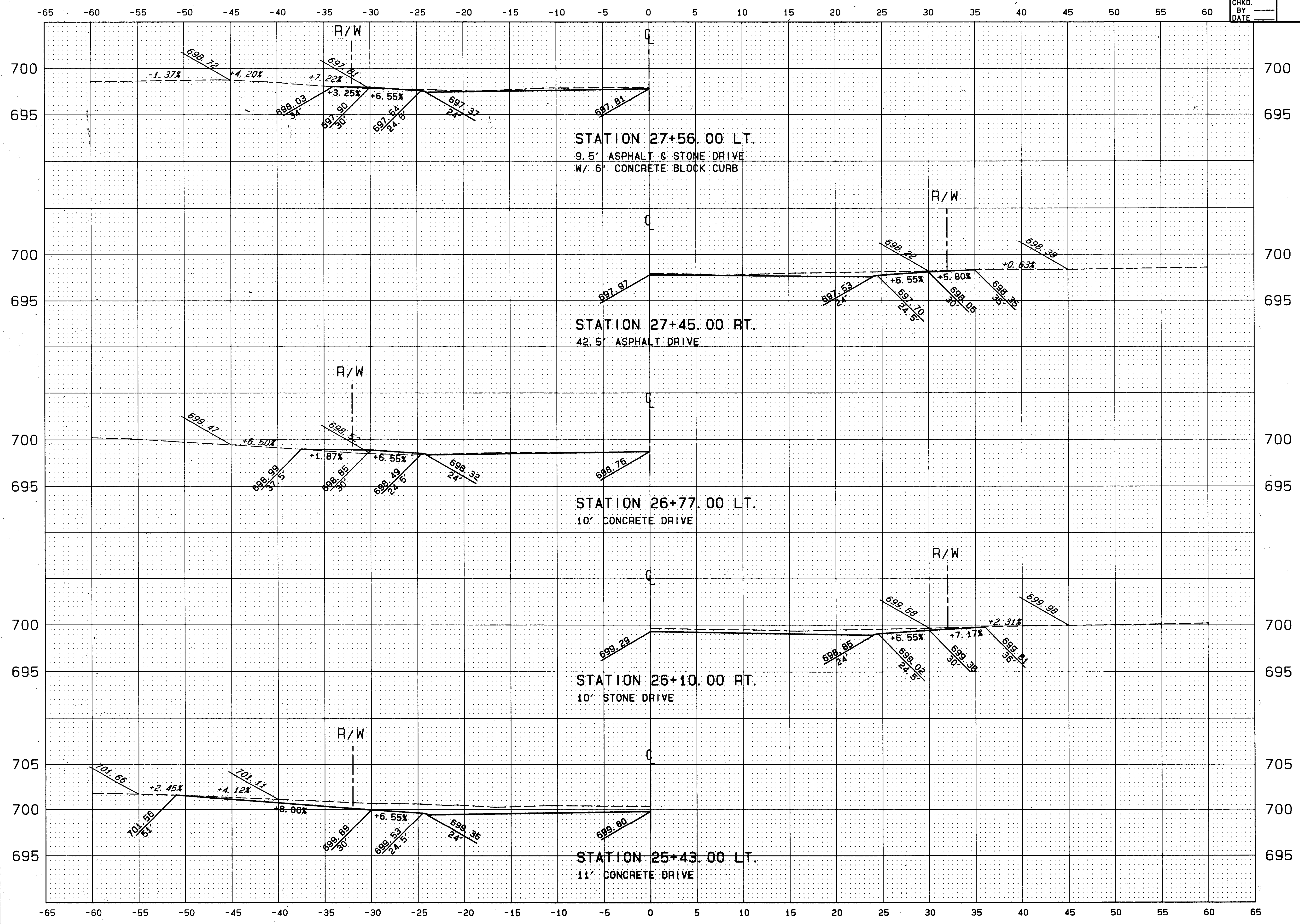
DRIVE PROFILES STA. 25+43 TO STA. 27+56
