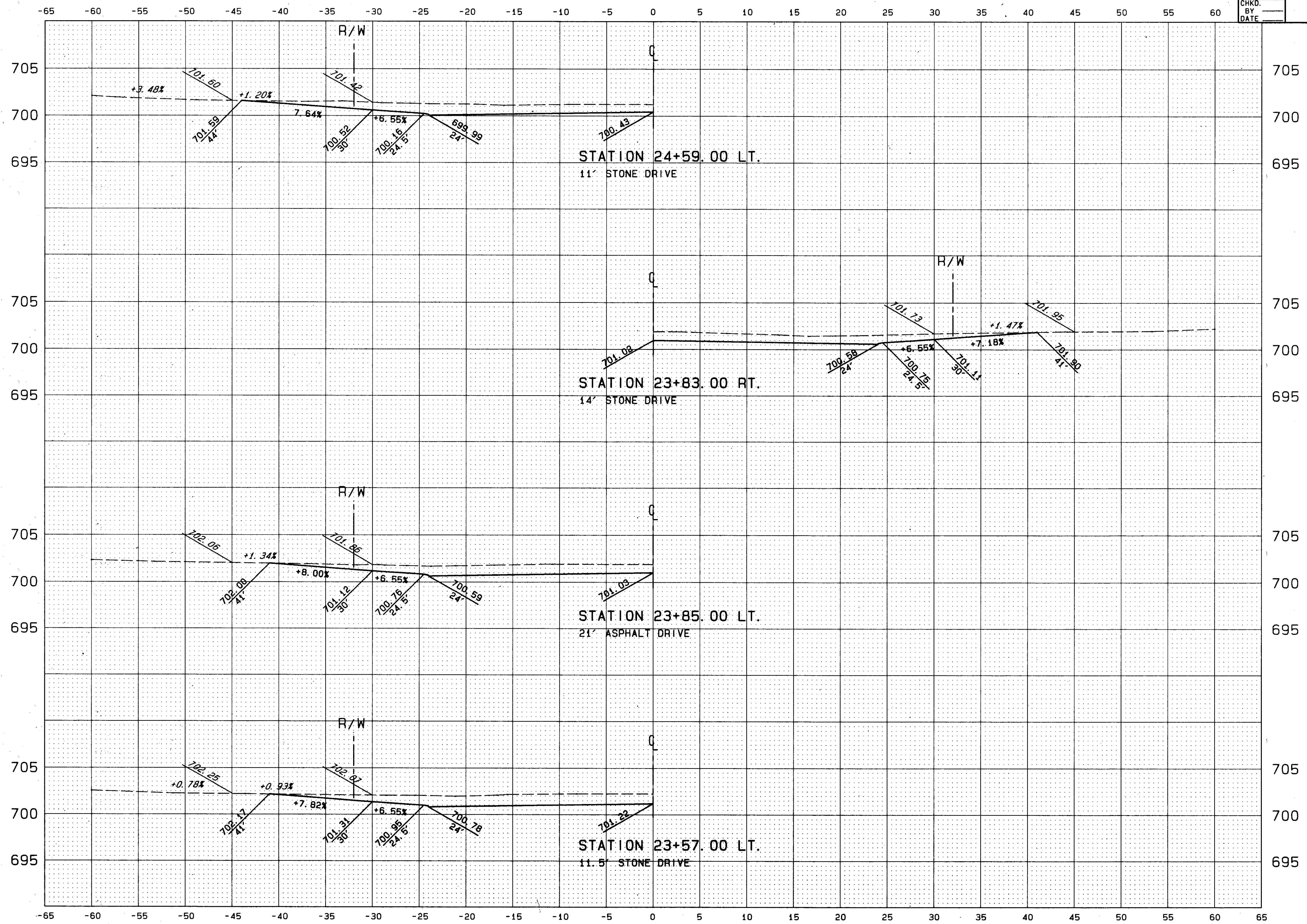
DRIVE PROFILES STA. 23+57 TO STA. 24+60
