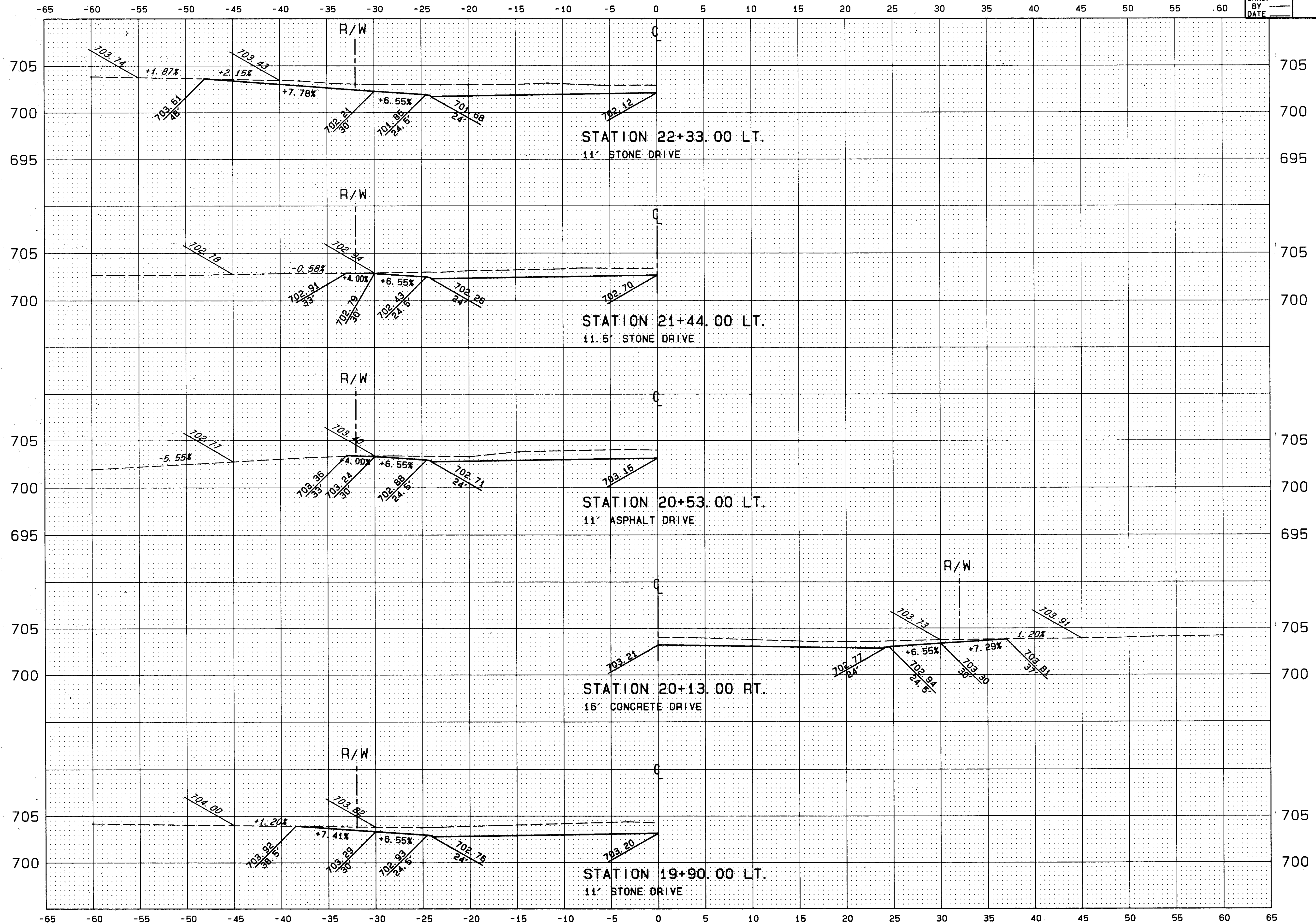
DRIVE PROFILES STA. 19+90 TO STA. 22+33
