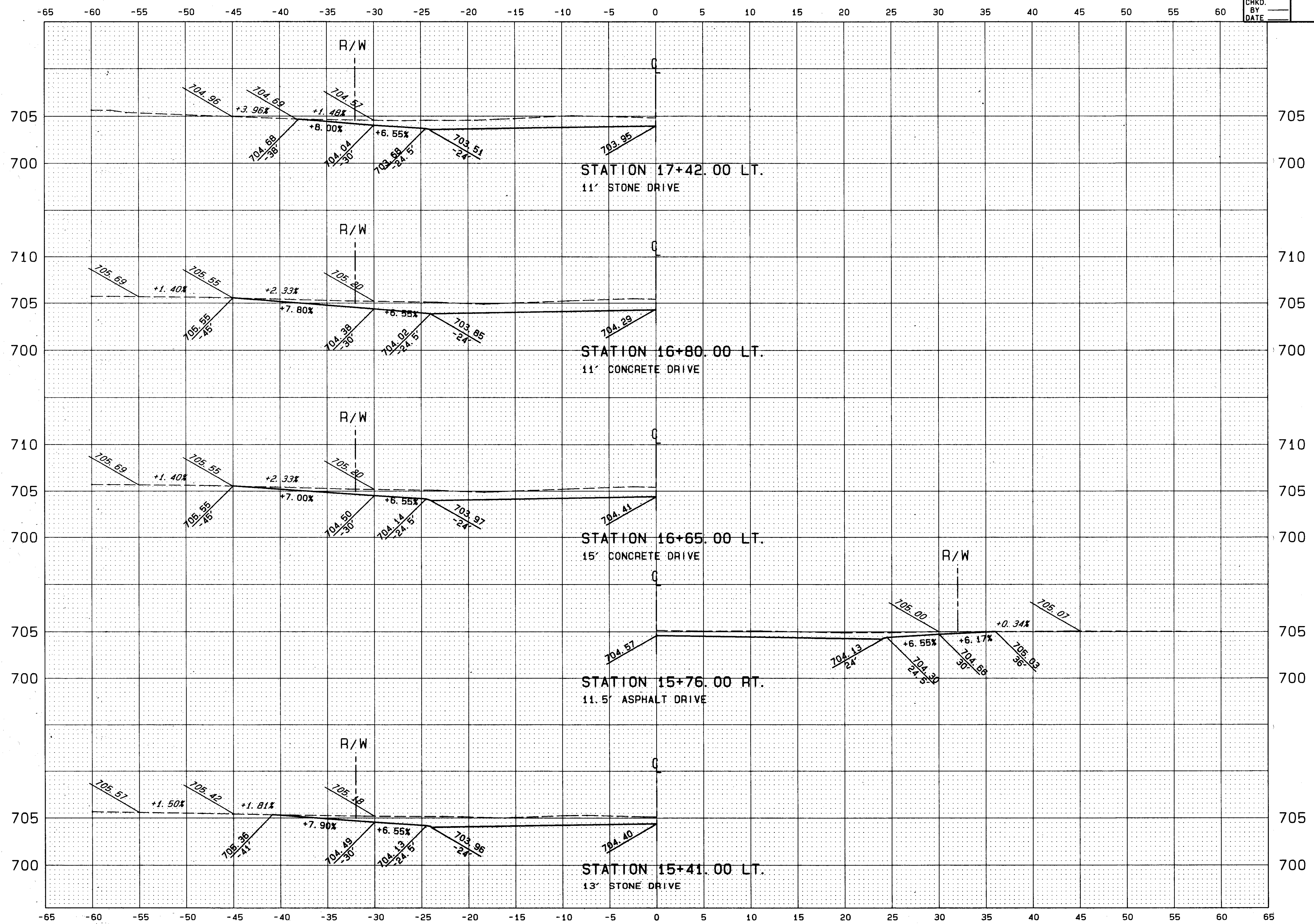
DRIVE PROFILES STA. 15+41 TO STA. 17+42
