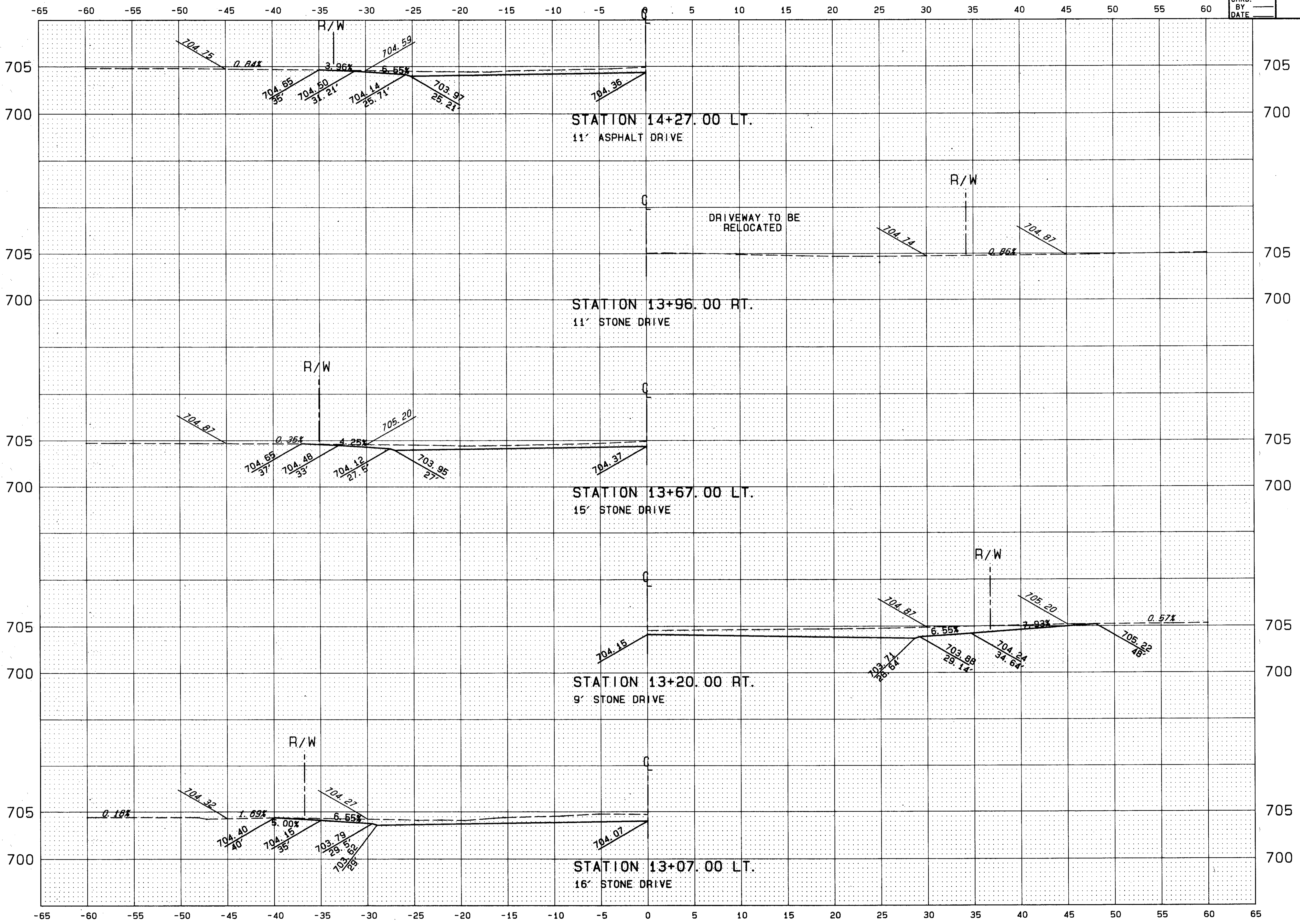
DRIVE PROFILES STA. 13+07 TO STA. 14+27
