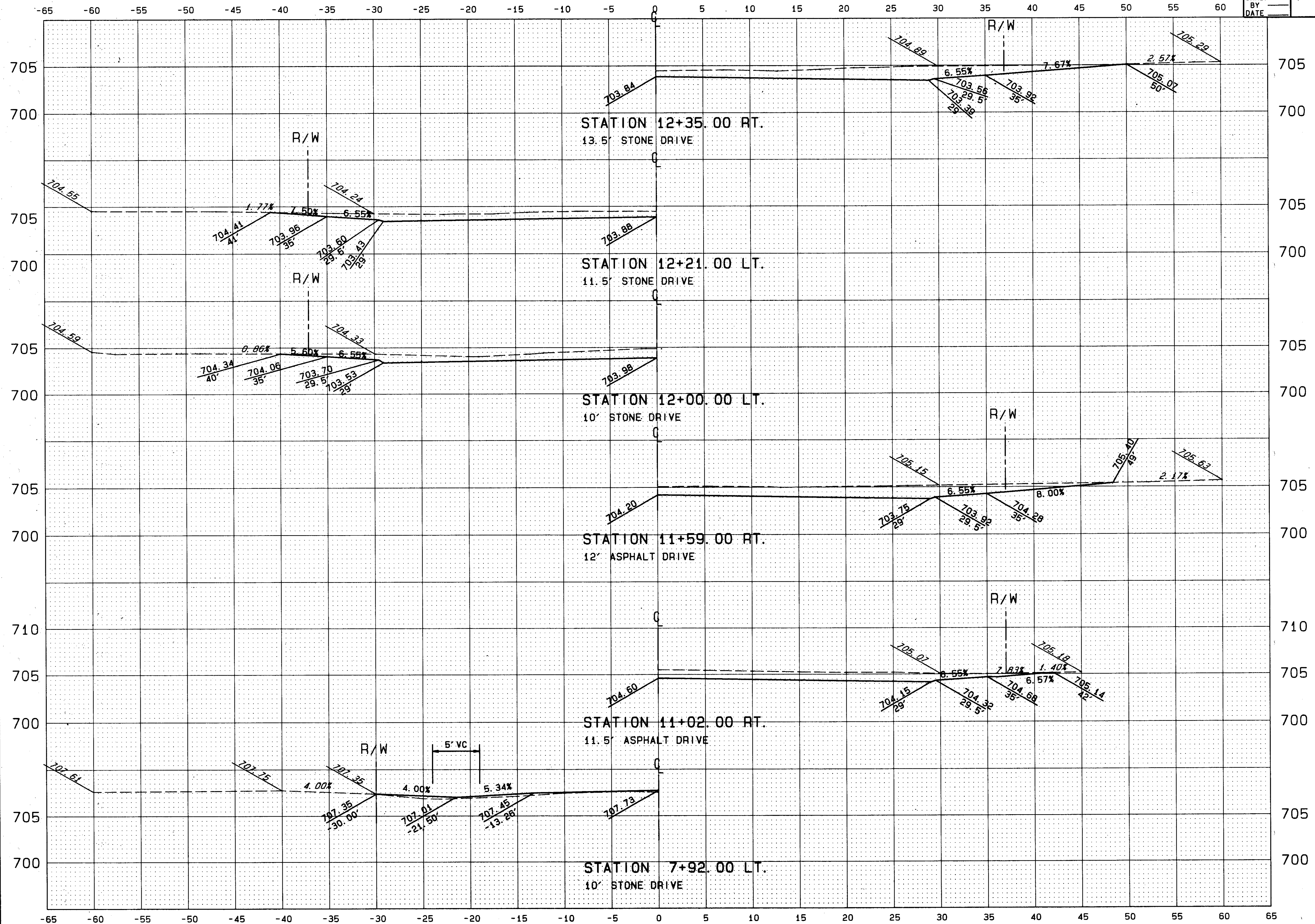
DRIVE PROFILES STA. 7+92 TO STA. 12+35
