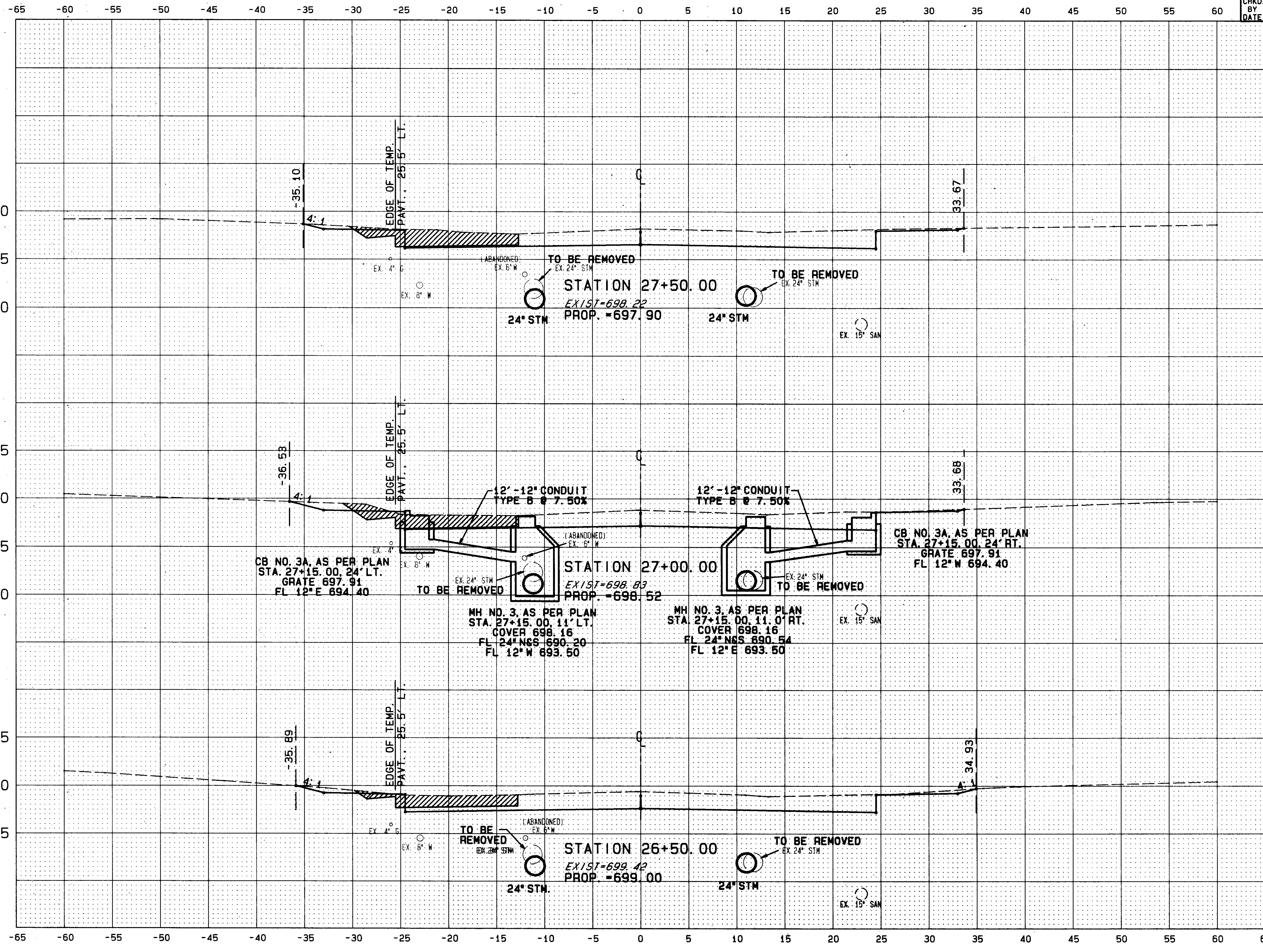
S. R. 615 CROSS SECTIONS STA. 26+50 TO STA. 27+50
