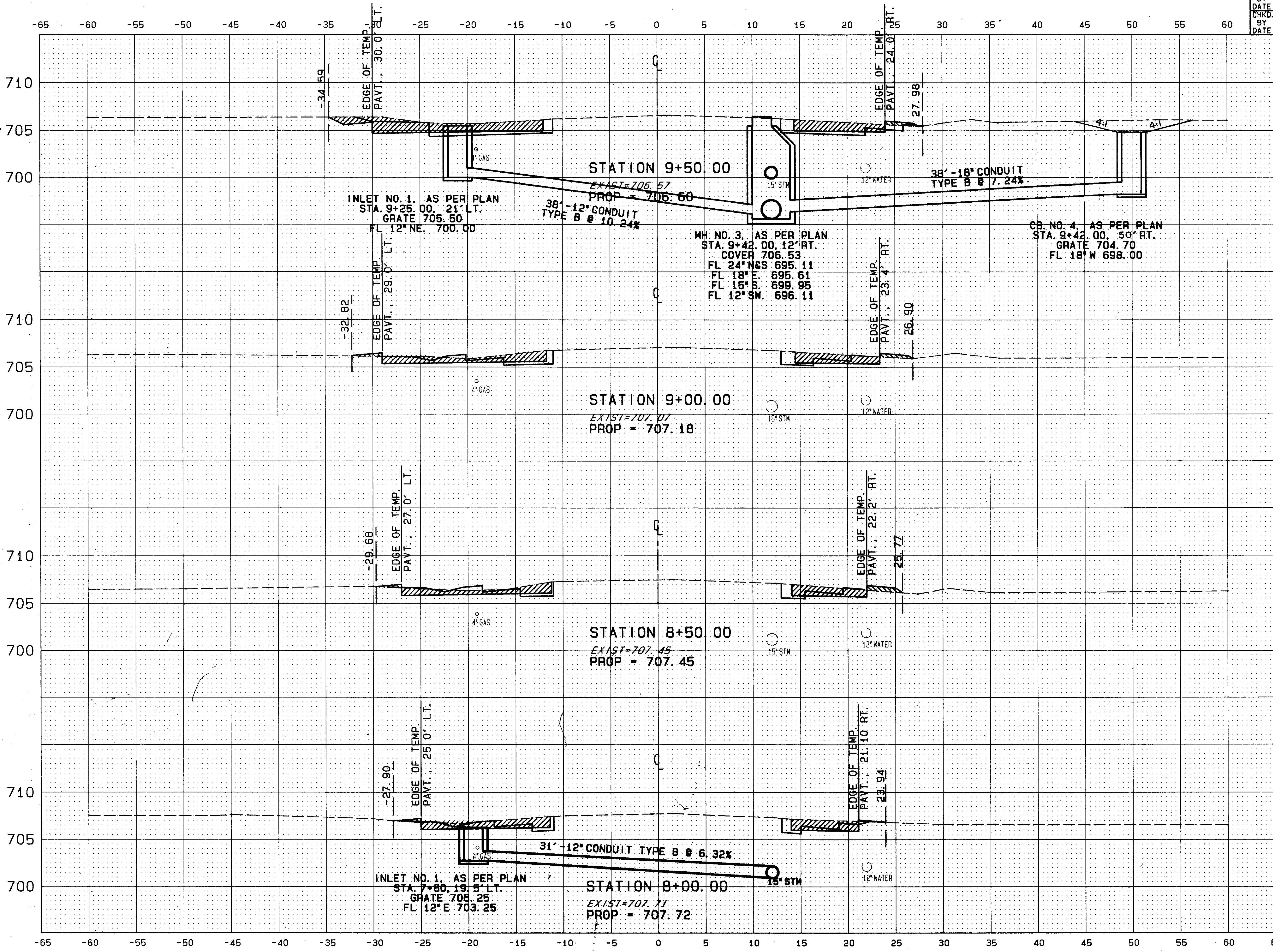
S. R. 615 CROSS SECTIONS STA. 8+00 TO STA. 9+50
