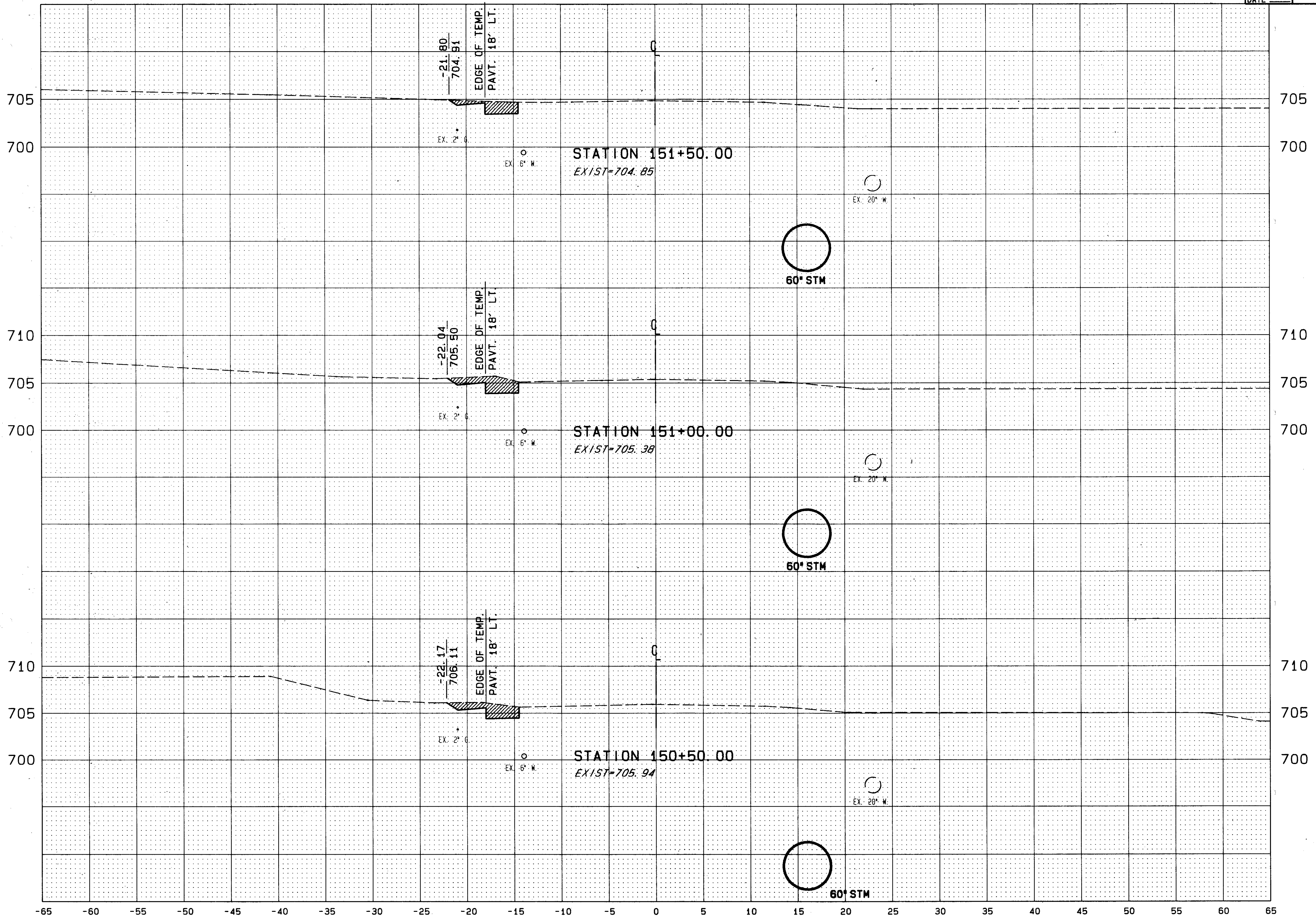
S. R. 84 CROSS SECTION STA. 150+50 TO STA. 151+50
