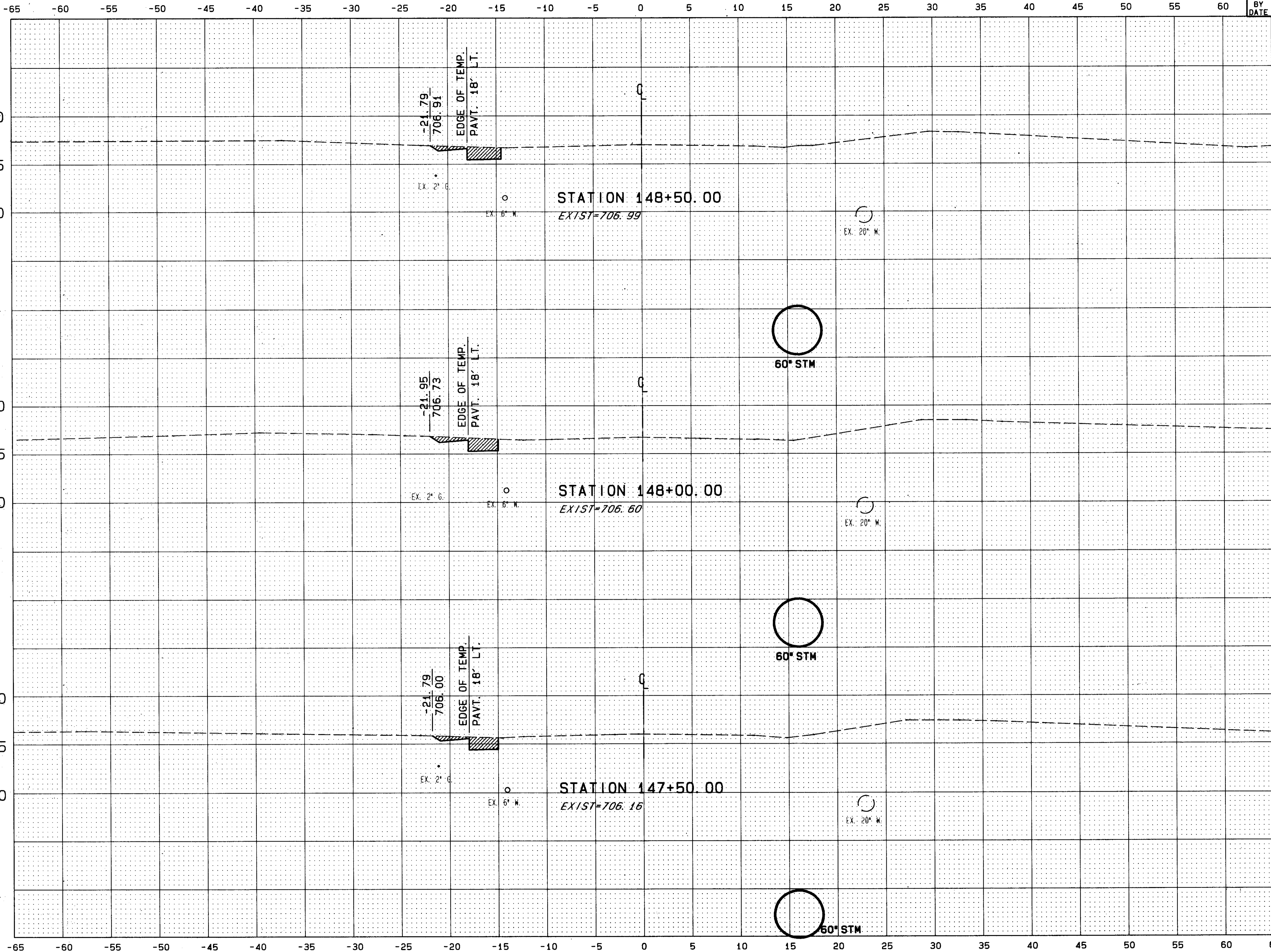
S. R. 84 CROSS SECTION STA. 147+50 TO STA. 148+50
