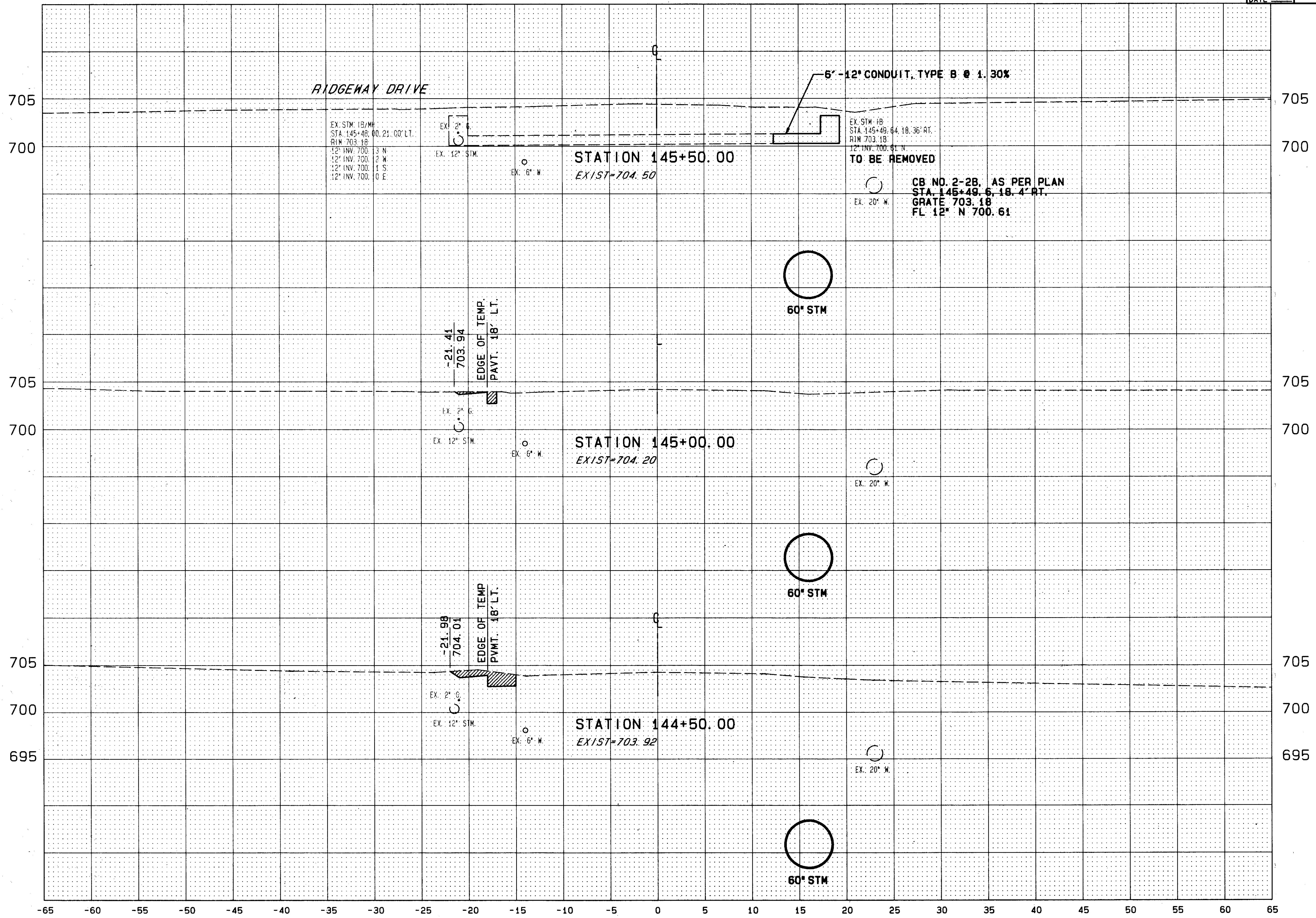
S. R. 84 CROSS SECTION STA. 144+50 TO STA. 145+50
