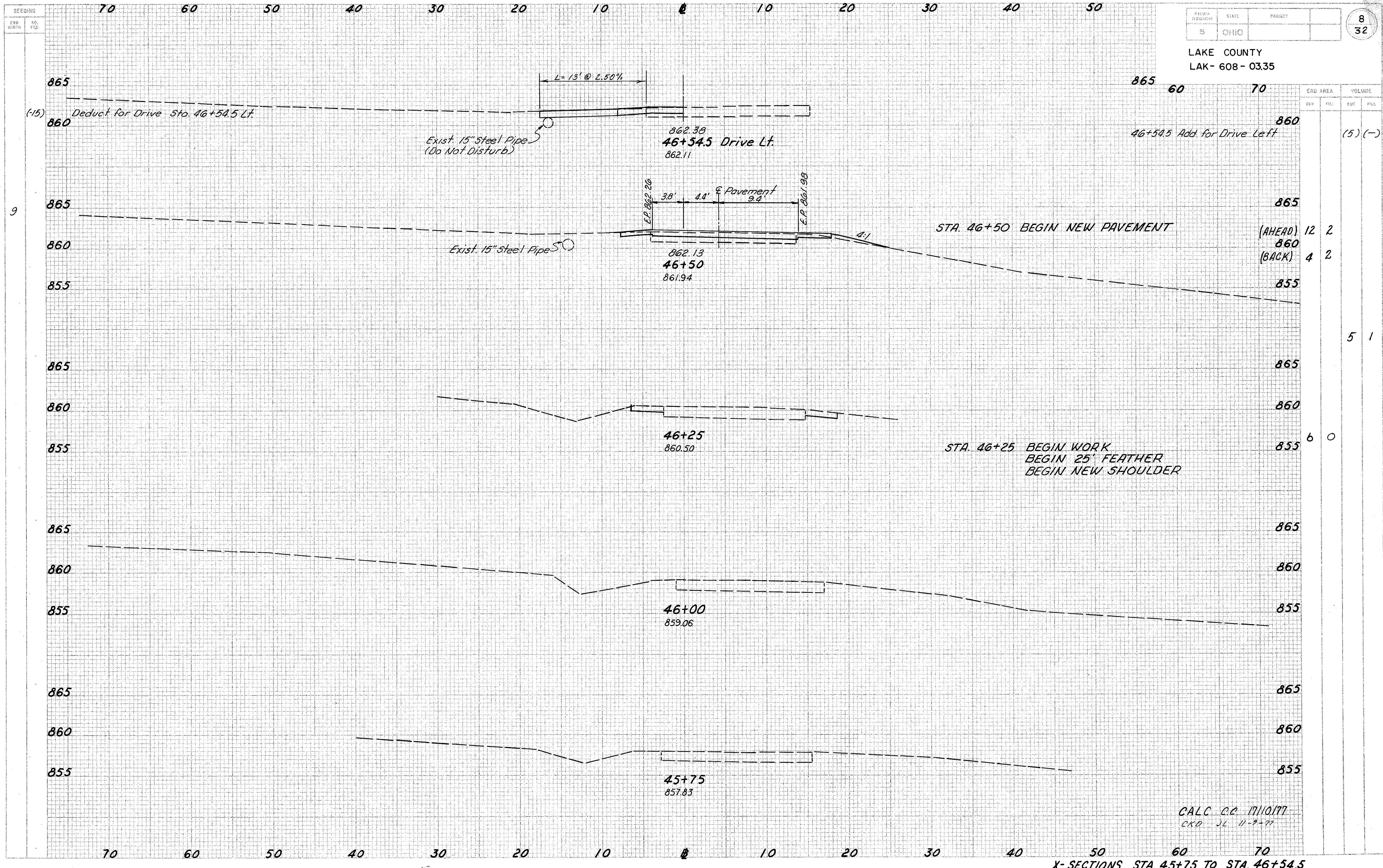
X-SECTIONS STA. 45+75 TO STA. 46+54.5
