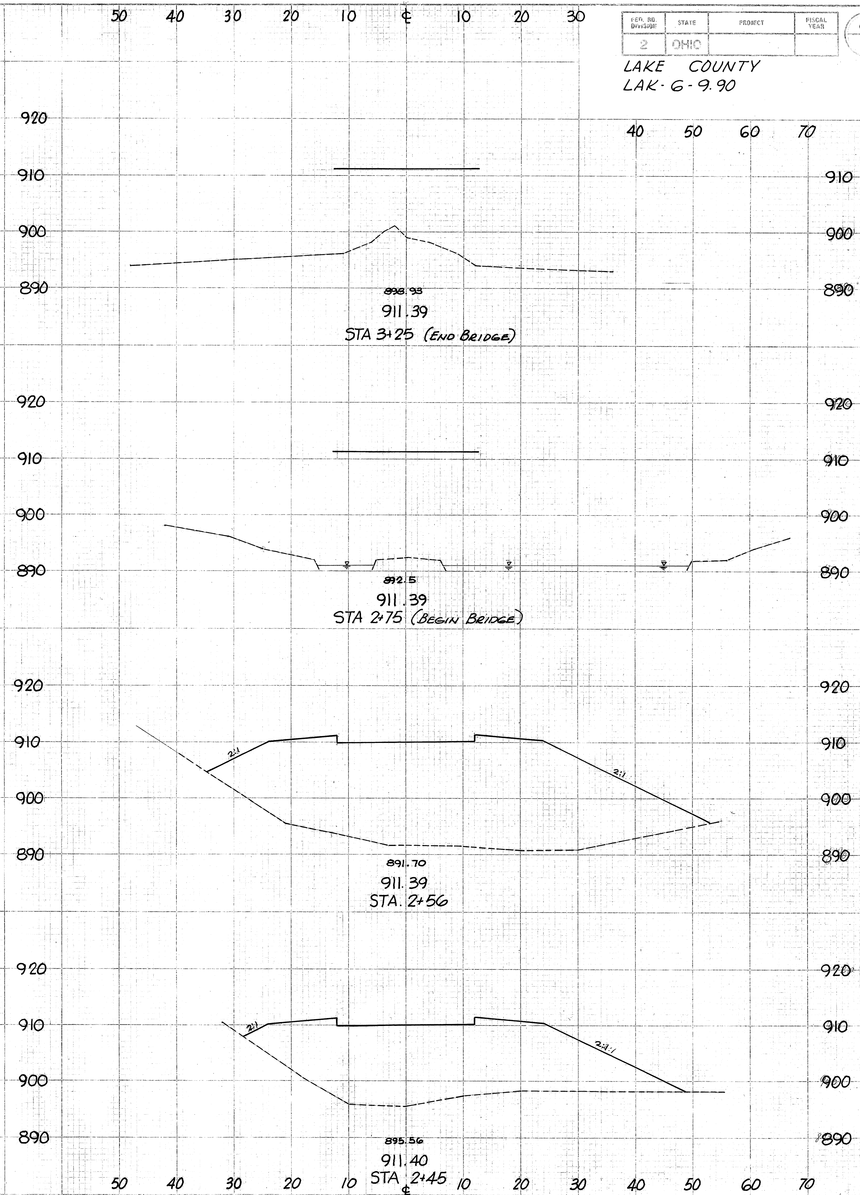
CROSS SECTIONS STA 524+75 to STA 3+25
