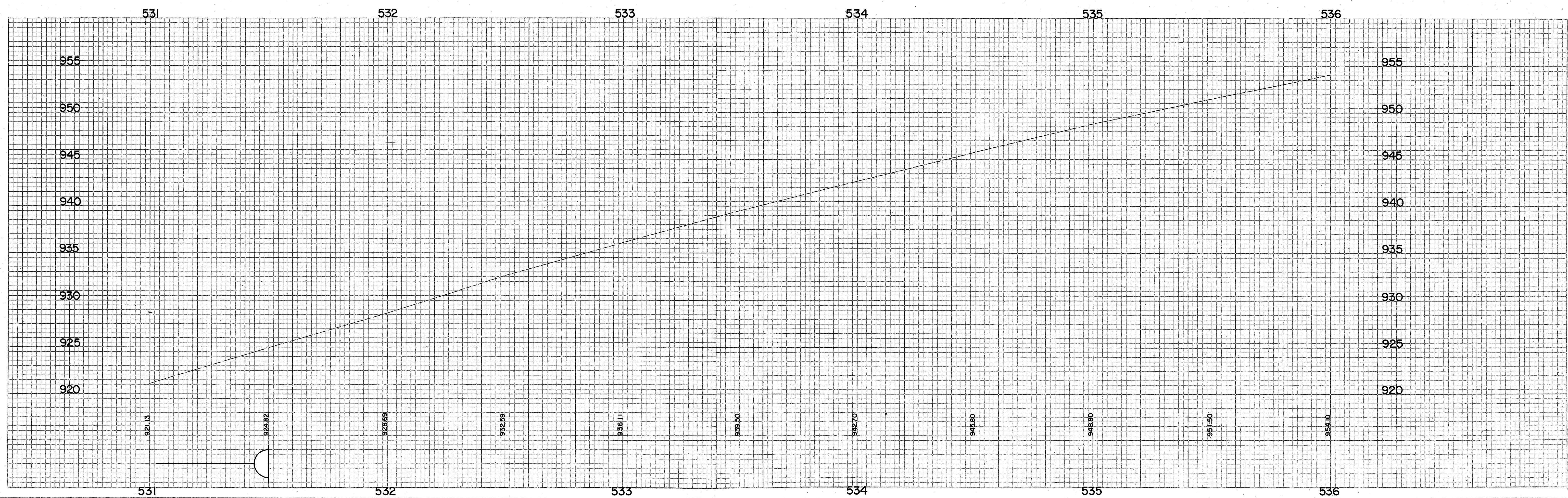
PLAN & PROFILE - P.R.C. STA. 531+02.43 (BACK) TO STA. 536+00
