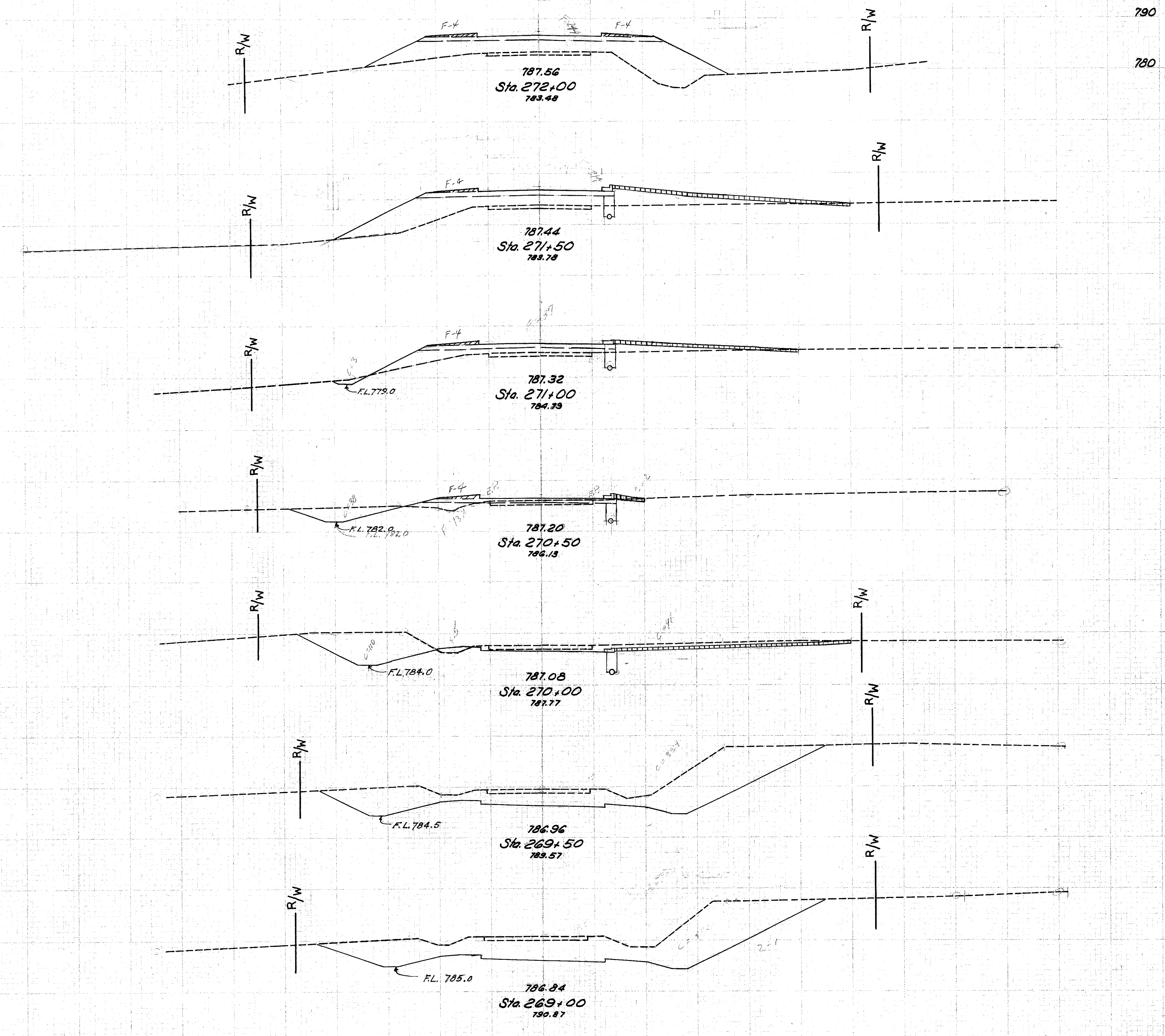
CROSS SECTIONS STA. 269+00 TO STA. 272+00
