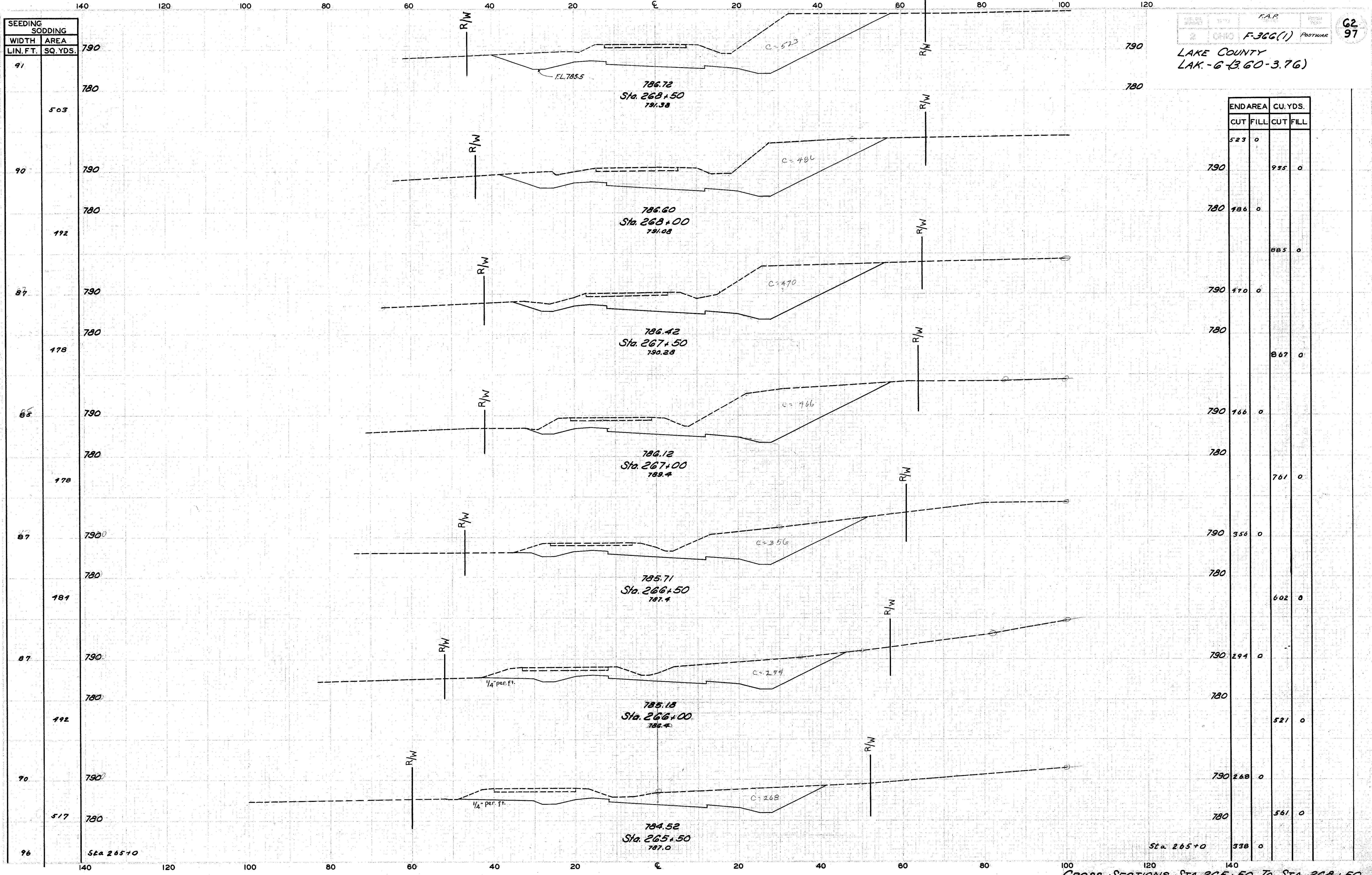
CROSS SECTIONS STA. 265+50 TO STA. 268+50
