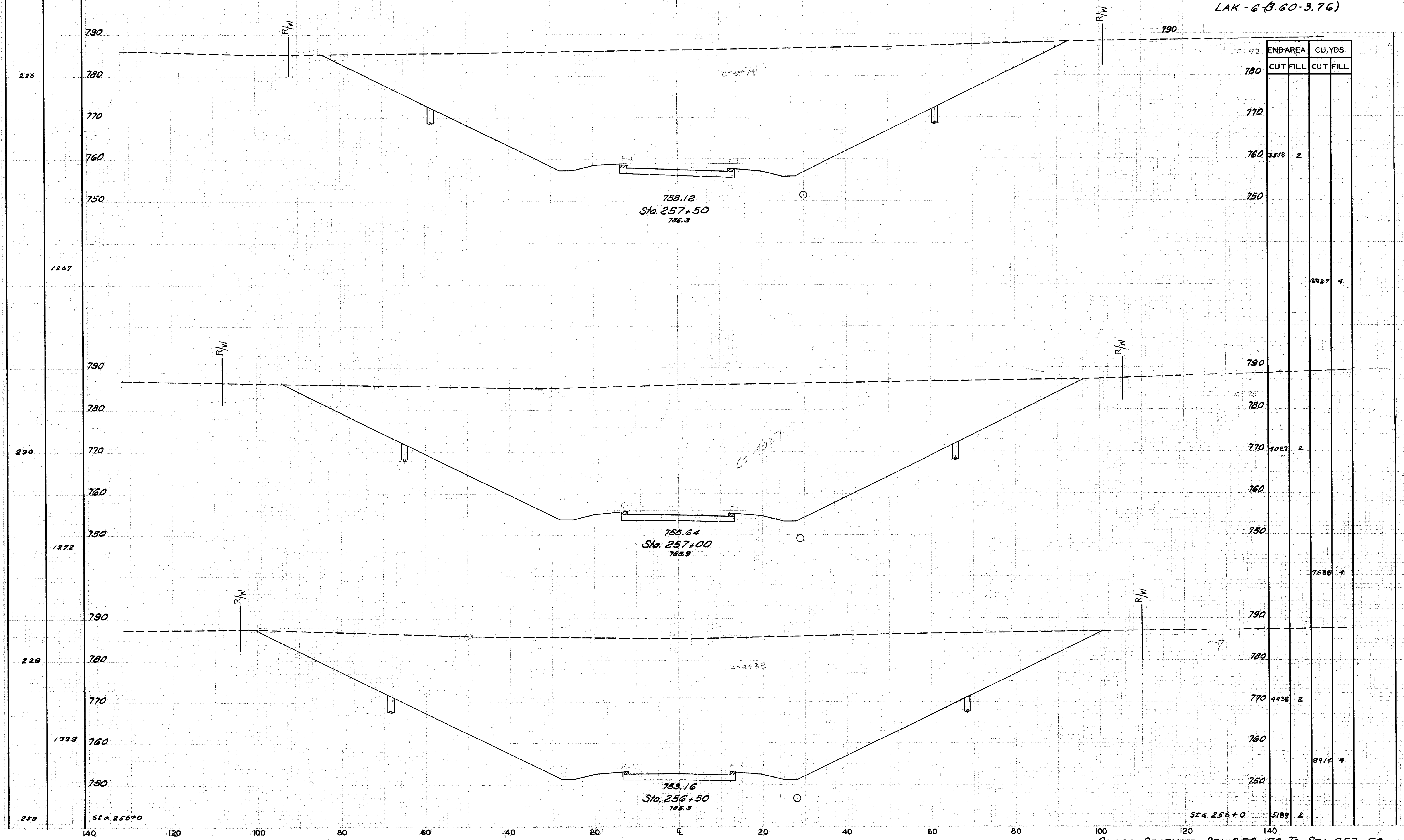
CROSS SECTIONS STA. 256+50 TO STA. 257+50
