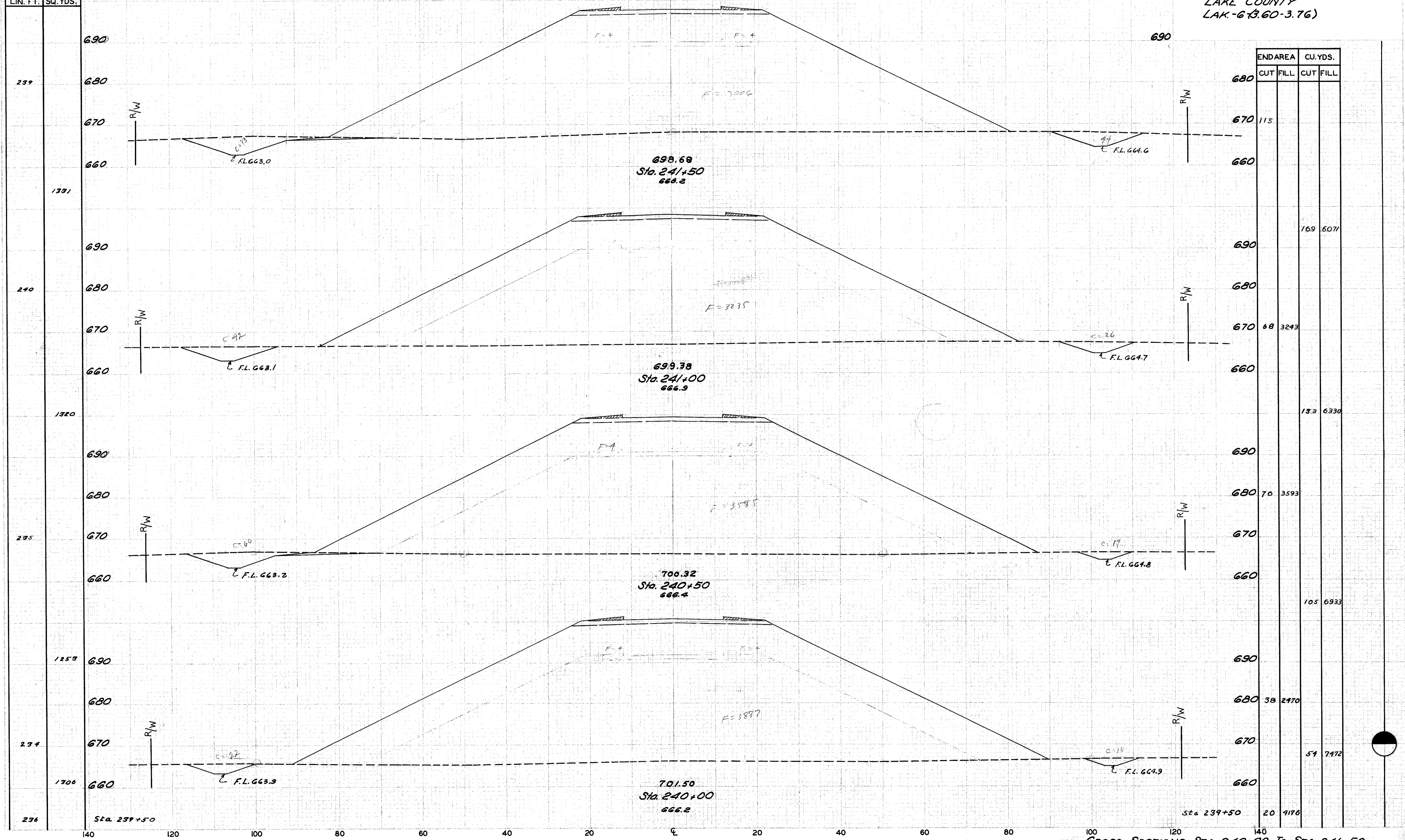
CROSS SECTIONS STA. 240+00 TO STA. 241+50
