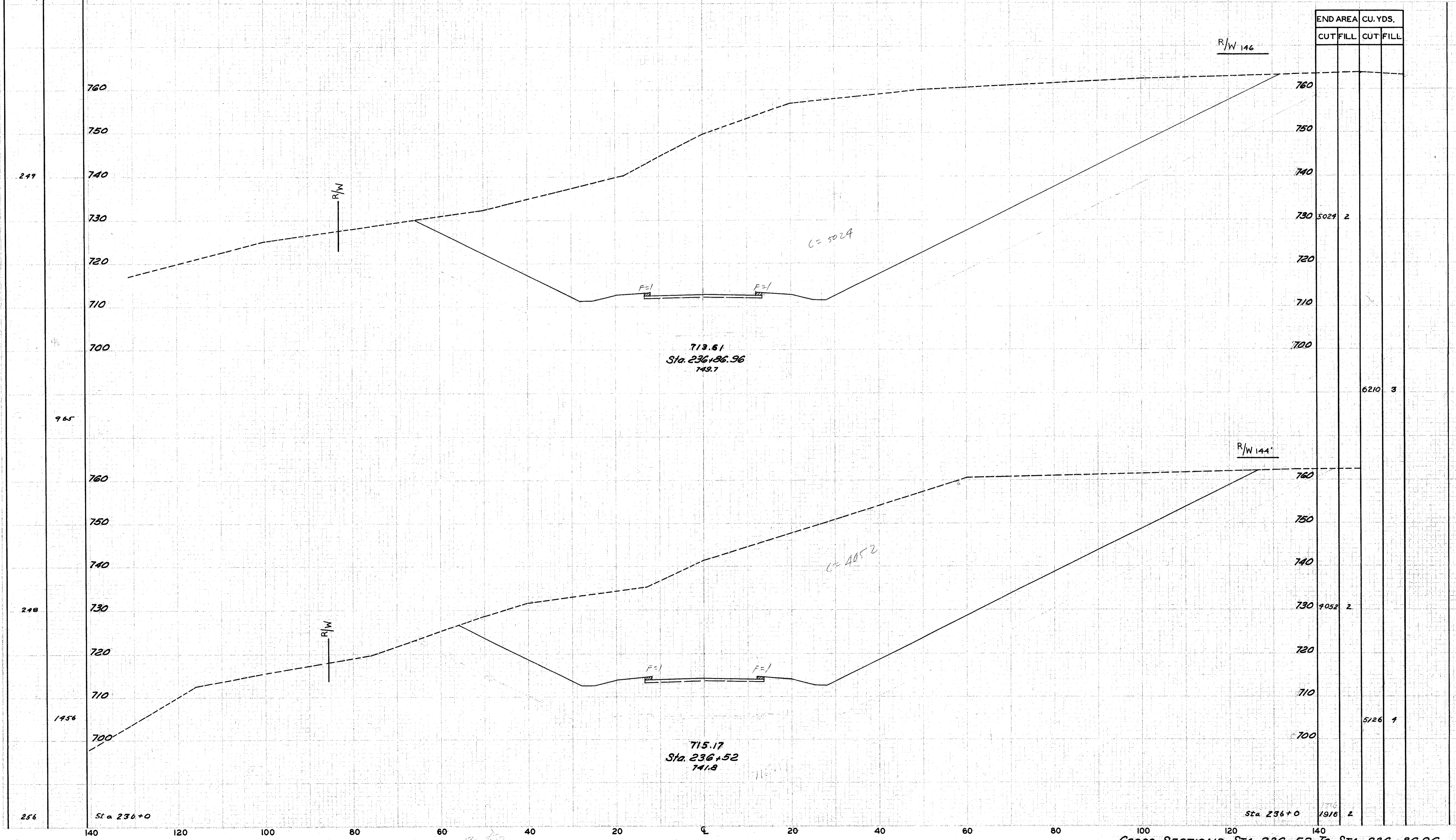
Cross SECTIONS STA. 236+52 TO STA. 236+86.96
