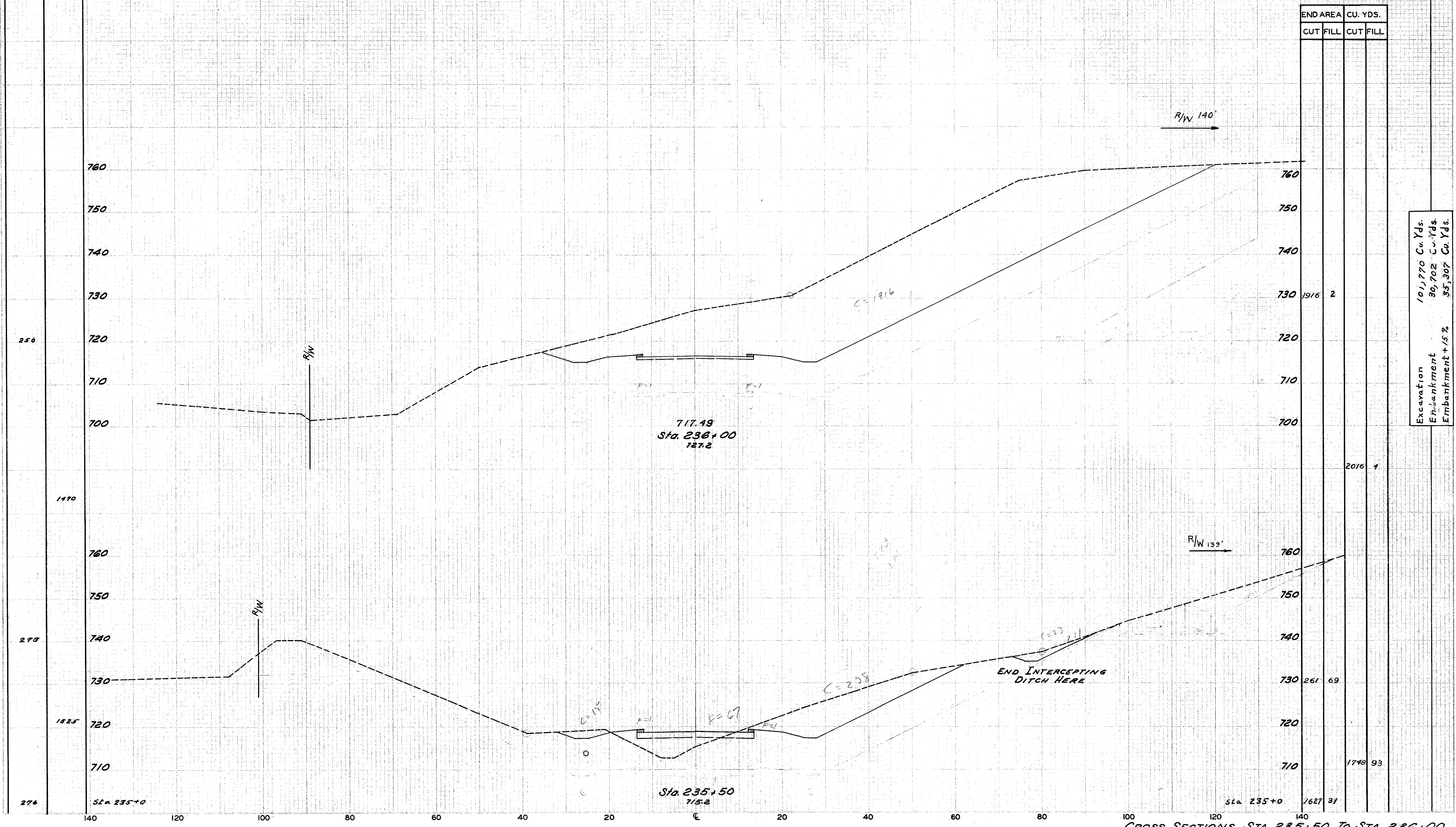
CROSS SECTIONS STA. 235+50 TO STA. 236+00
