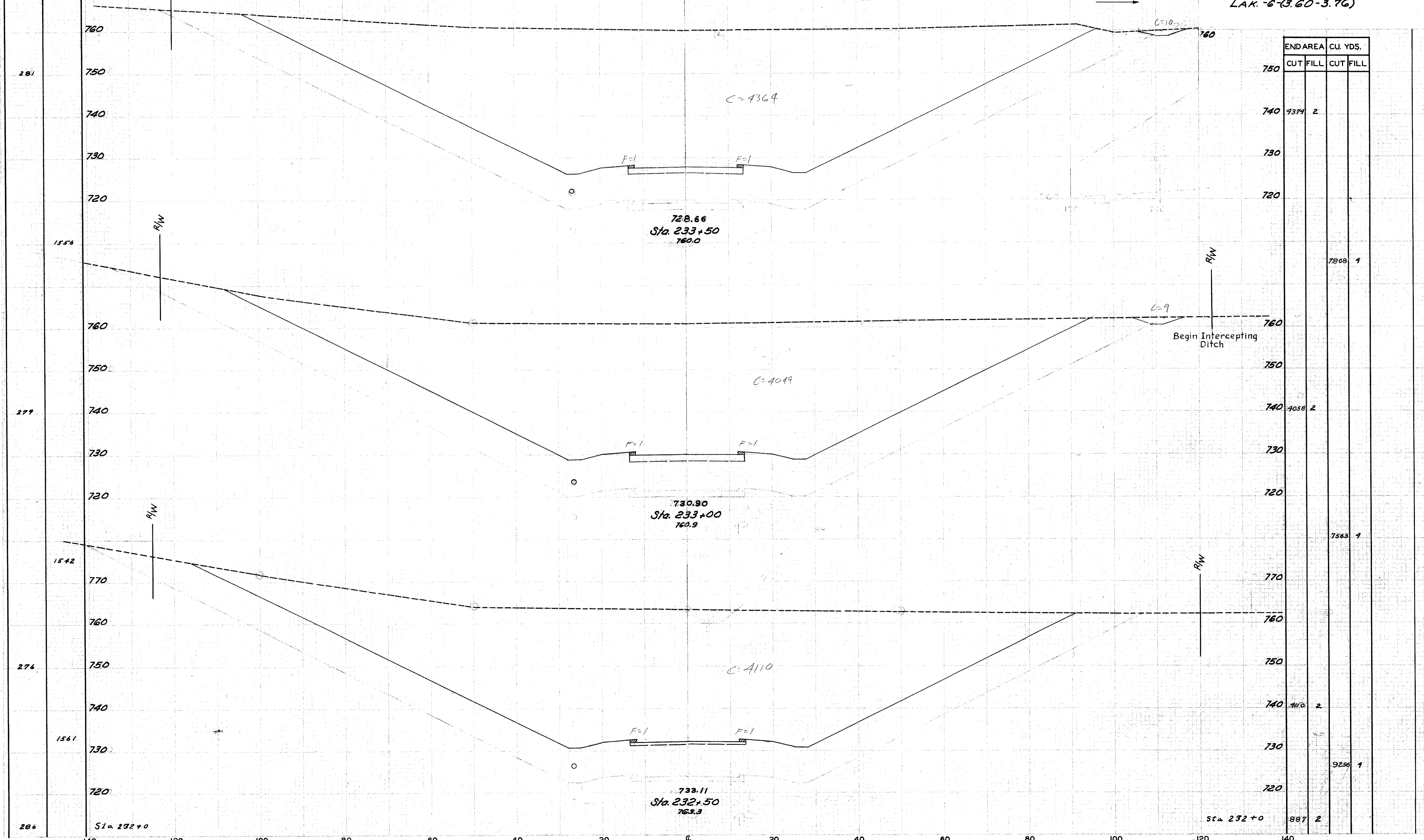
CROSS SECTIONS STA. 232+50 TO STA. 233+50
