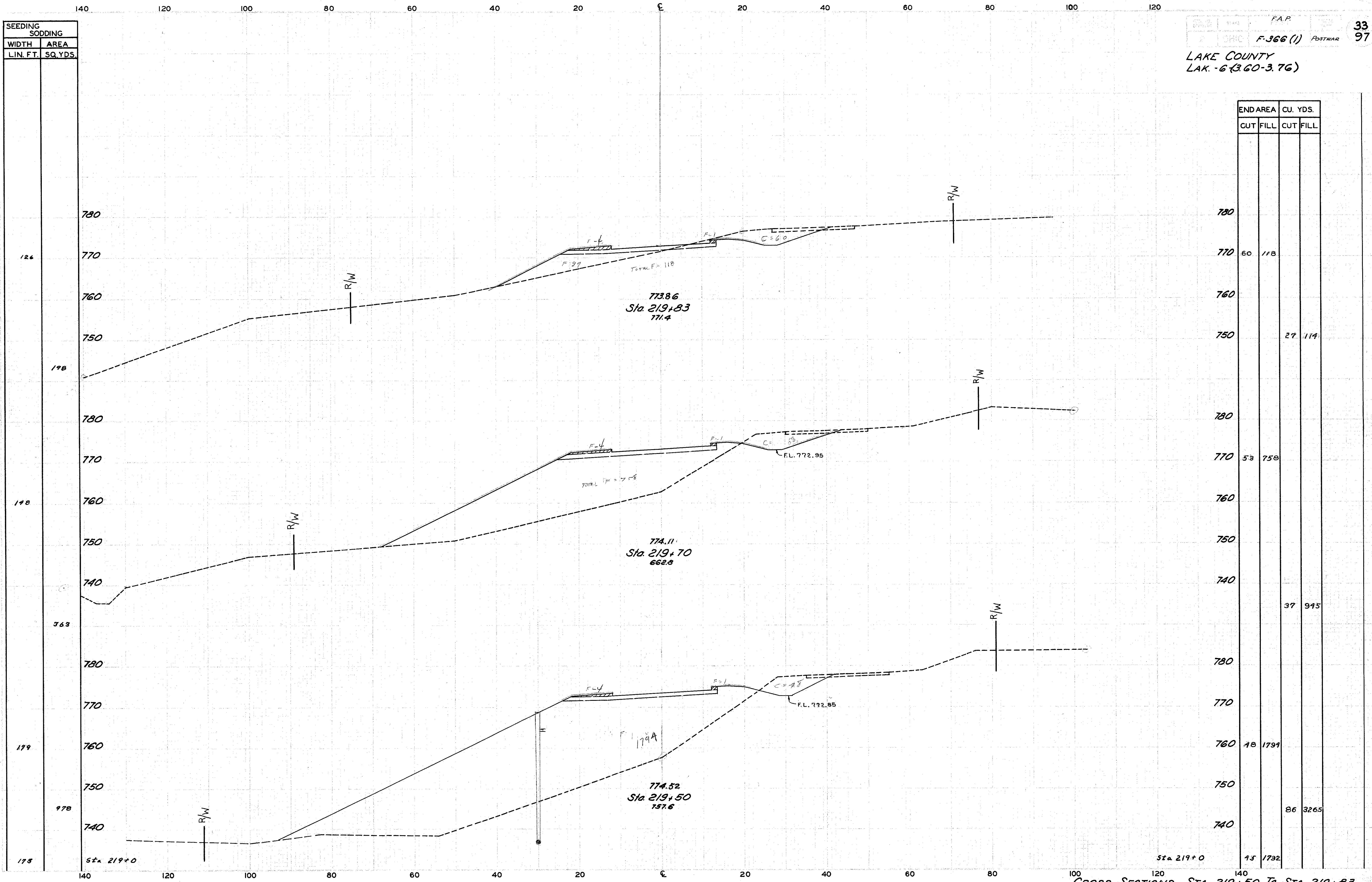
Cross Sections STA. 219+50 To STA. 219+83
