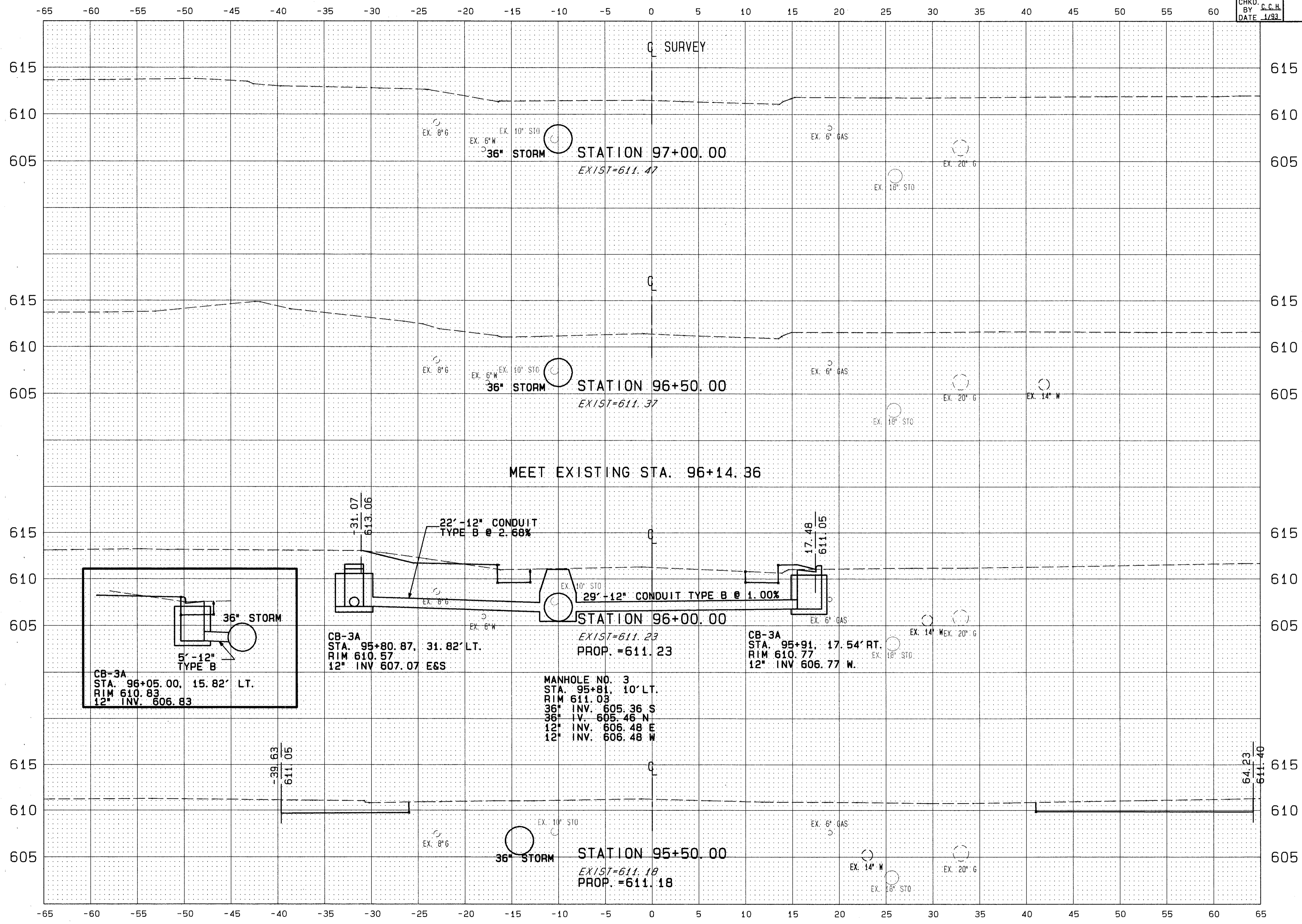
CROSS SECTION STA. 95+50 TO STA. 97+00
