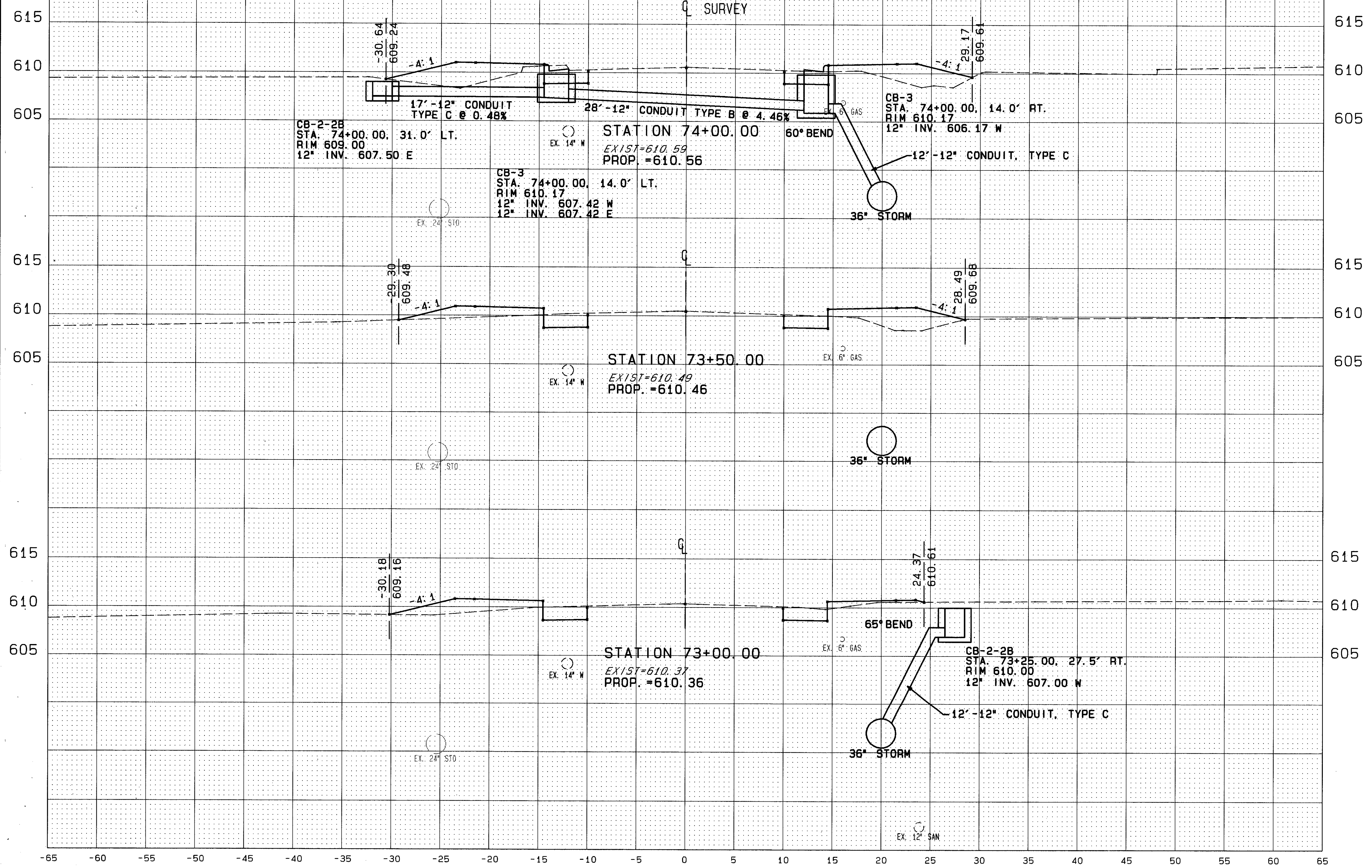
CROSS SECTION STA. 73+00 TO STA. 74+00
