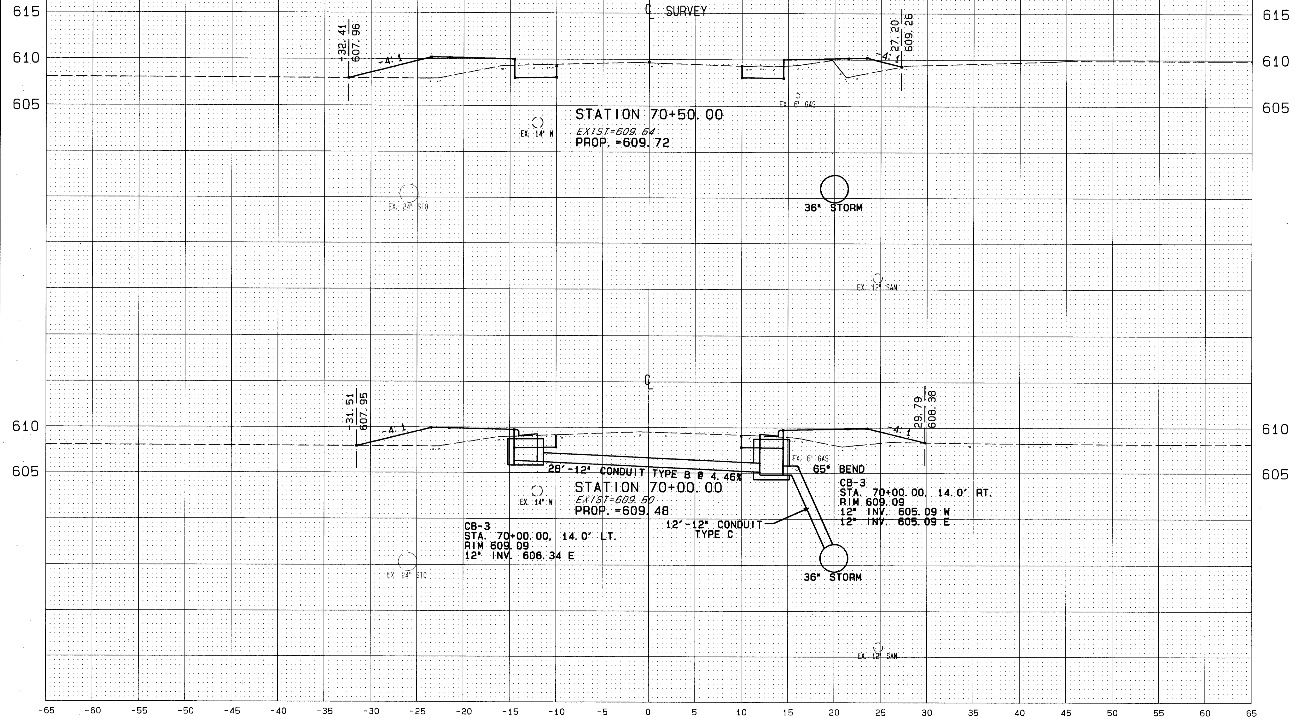
CROSS SECTION STA. 70+00 to STA. 70+50
