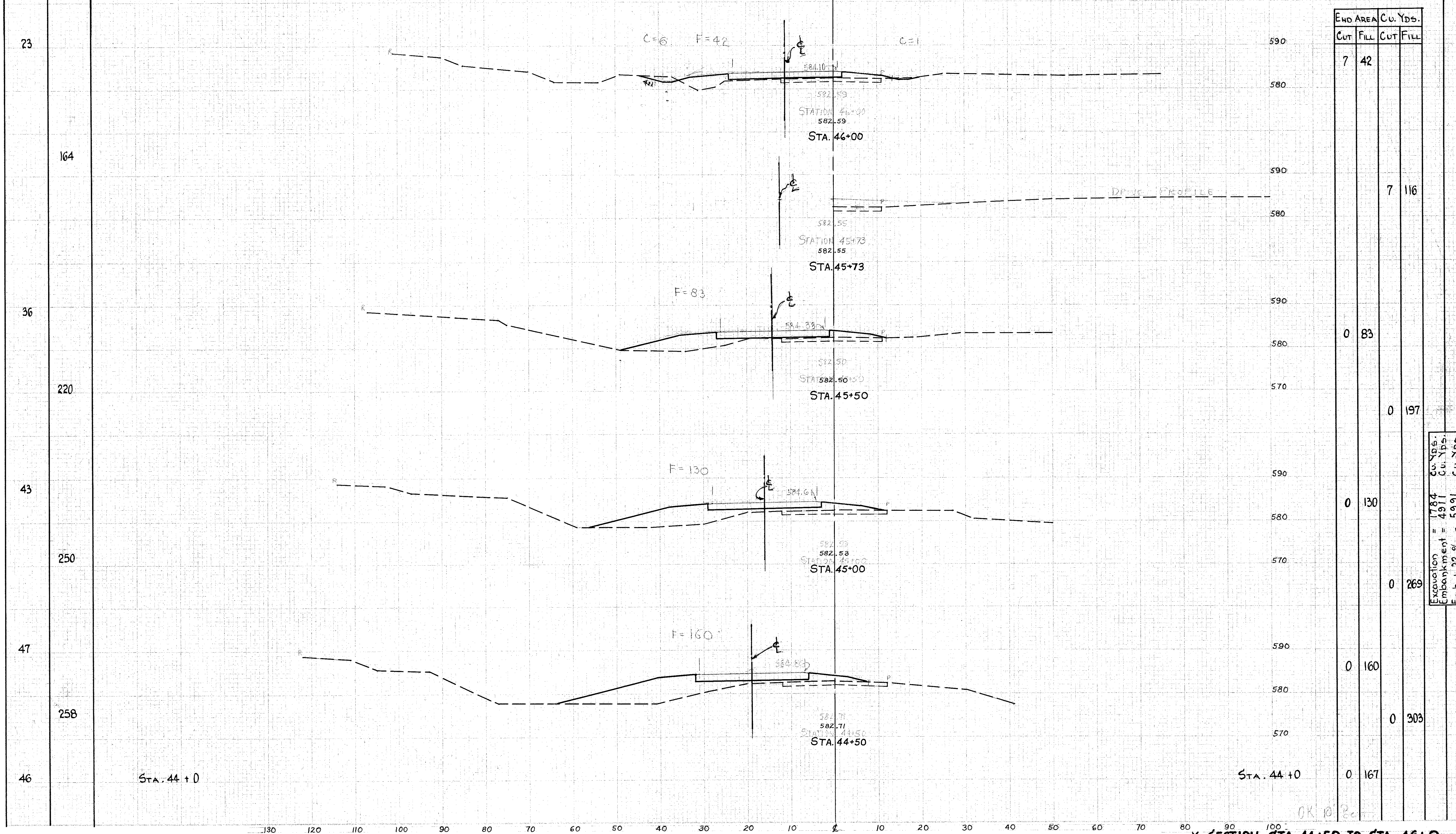
X-SECTION STA. 44+50 TO STA. 46+00
