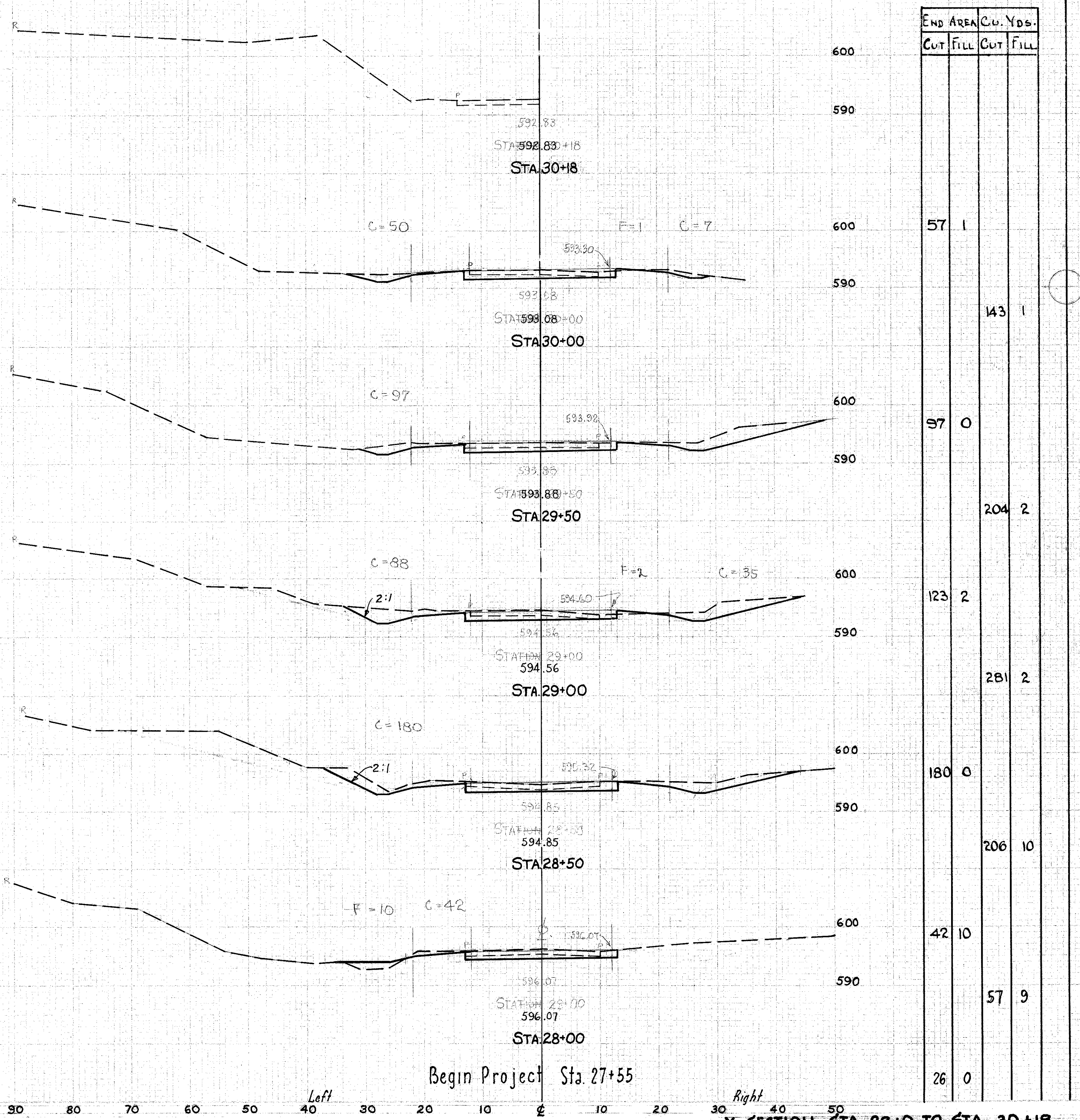
X-SECTION STA. 28+0 TO STA. 30+18
