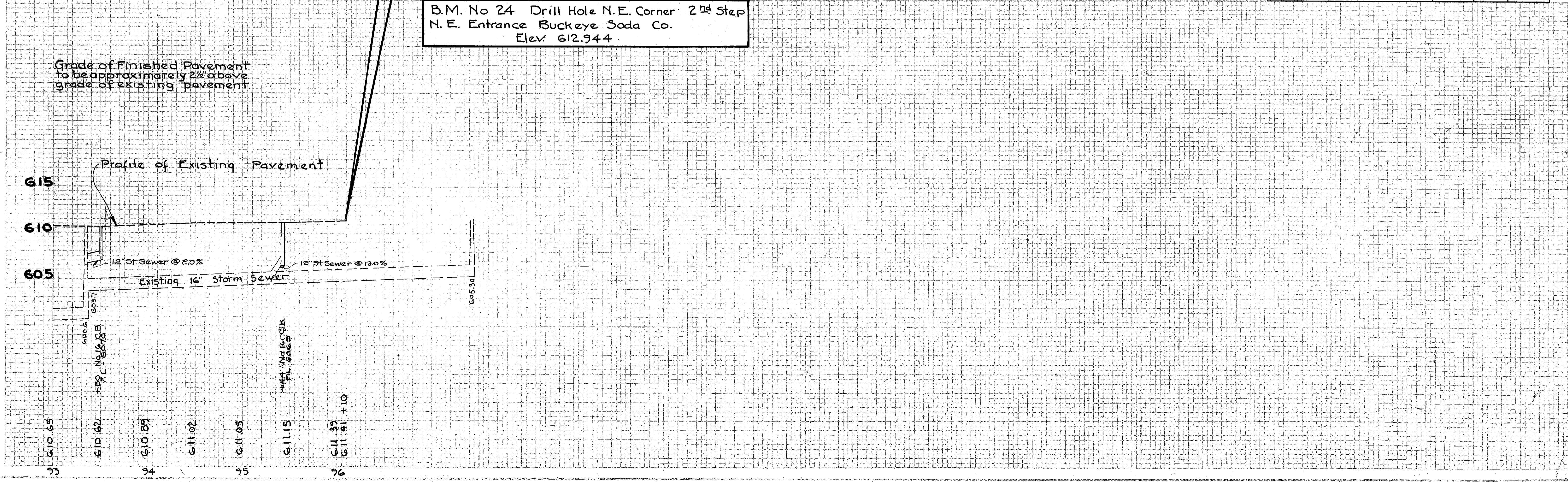
PLAN & PROFILE STA. 93+00 TO STA. 102+00
