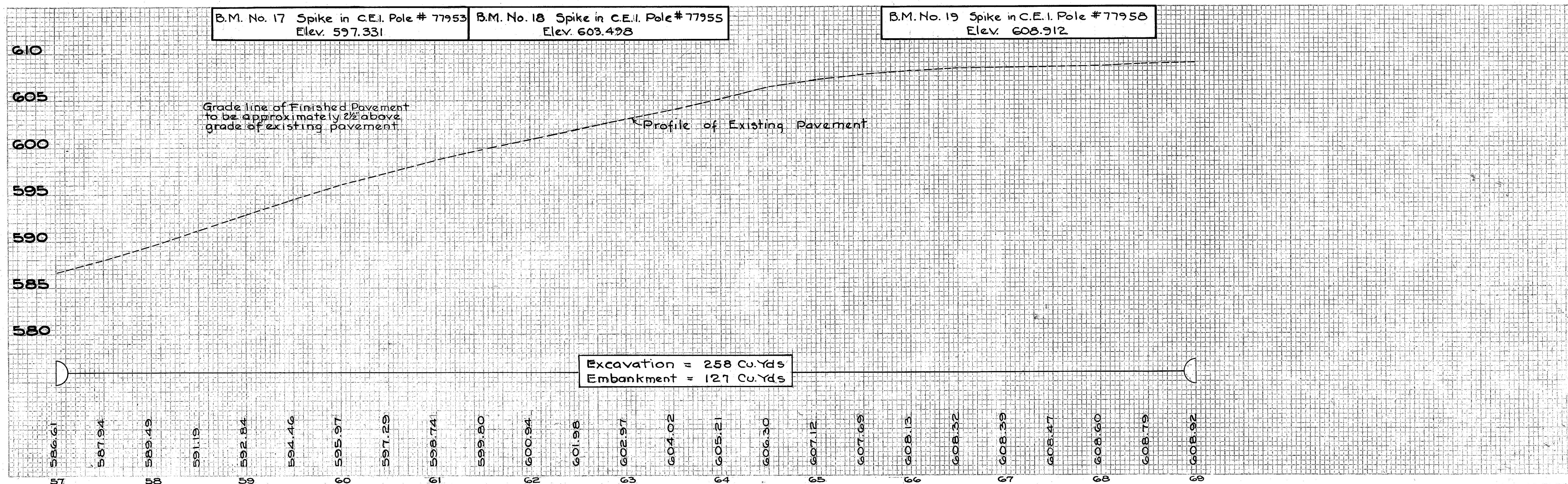
PLAN & PROFILE STA. 57+00 TO STA. 69+00
