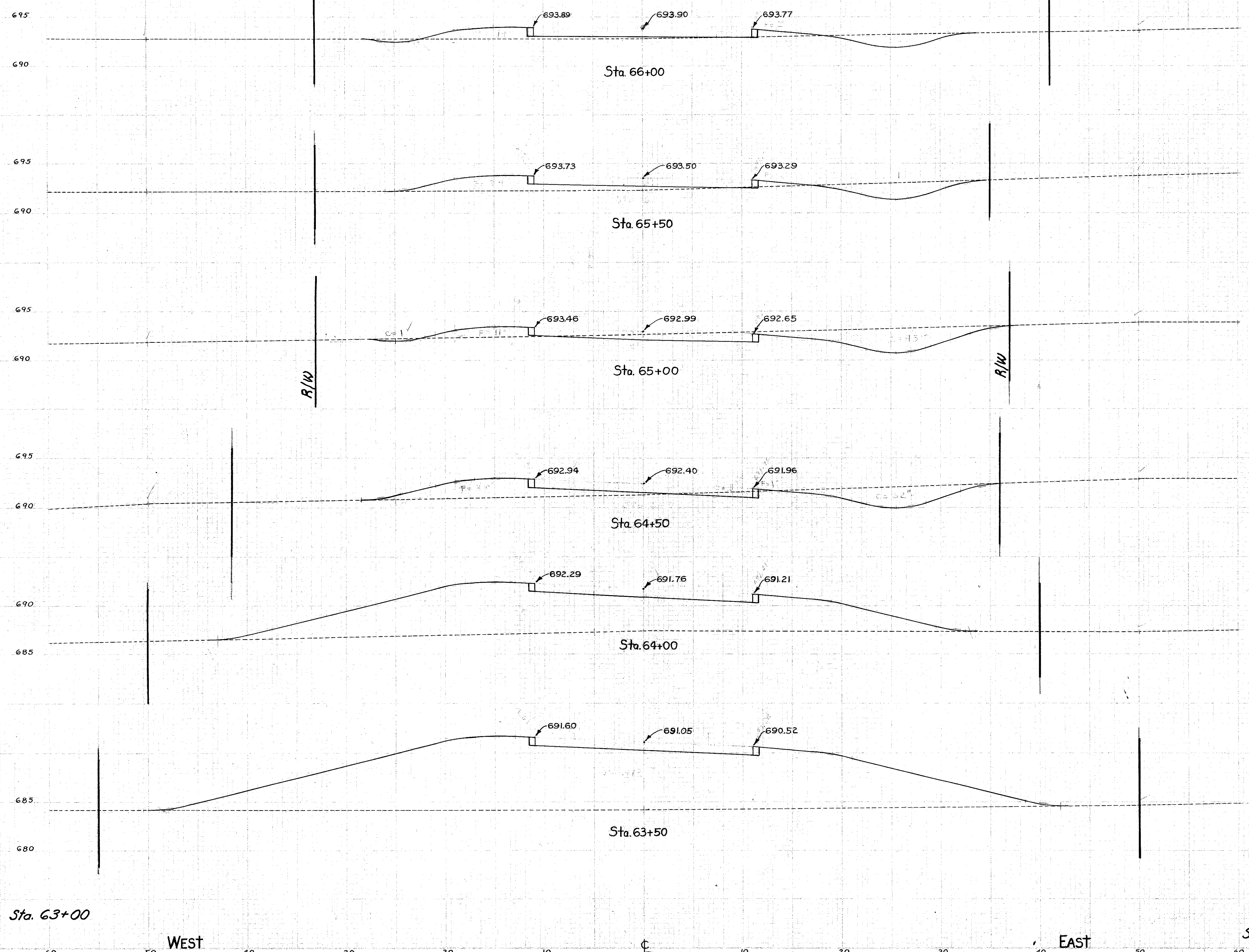
CROSS SECTIONS STA. 63+50 TO STA. 66+00
