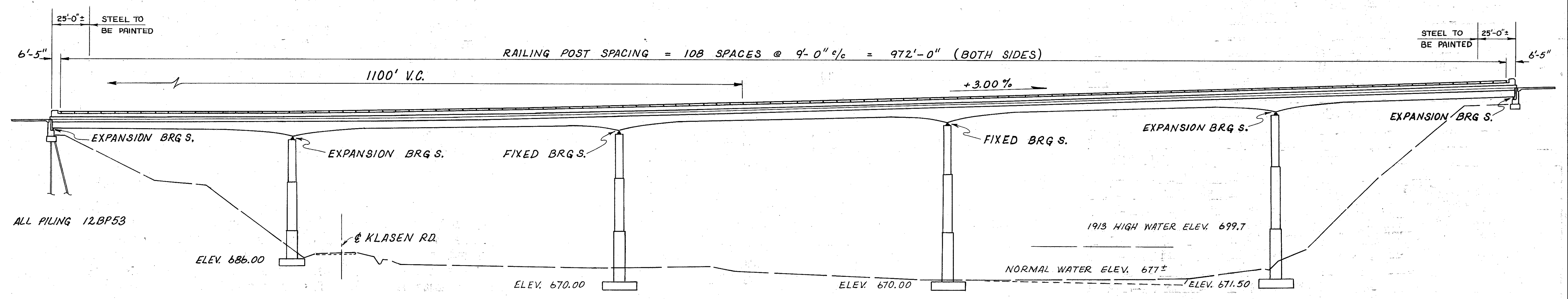
ELEVATION
