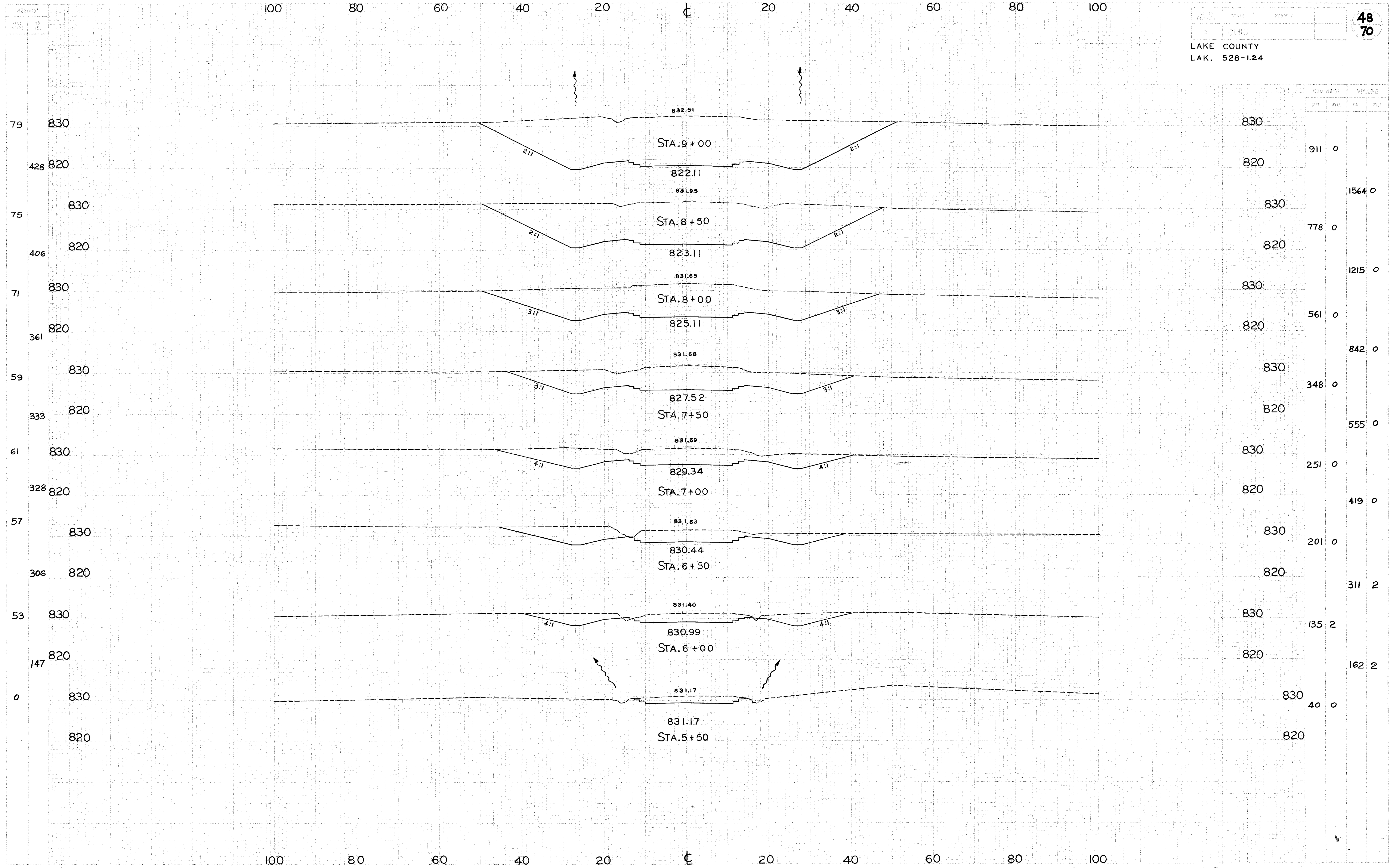
S.R. 307 ... CROSS SECTIONS ... STA. 5+50 TO STA. 9+00
