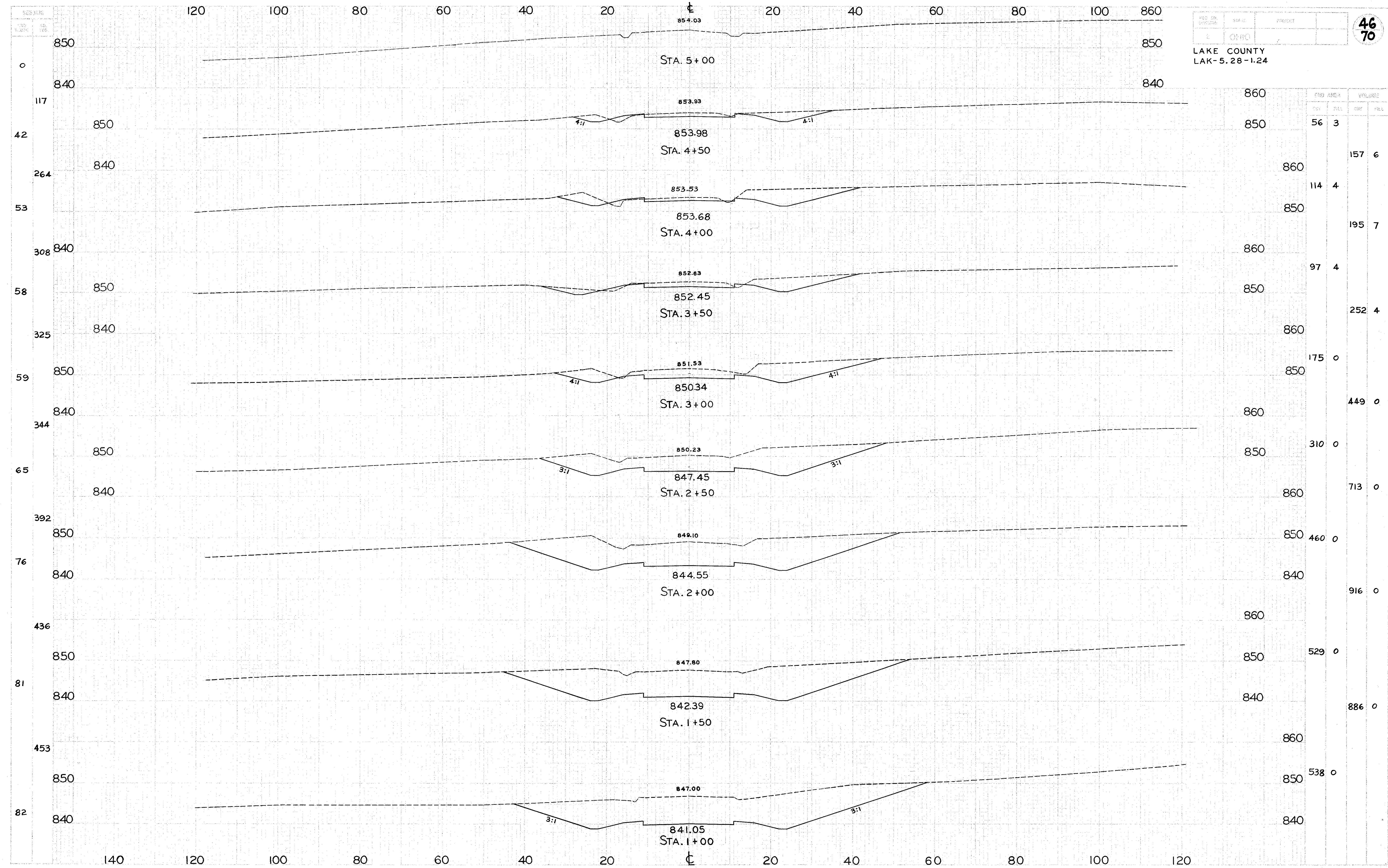
GRISWOLD ROAD... CROSS SECTIONS... STA. 1+00 TO STA. 5+00
