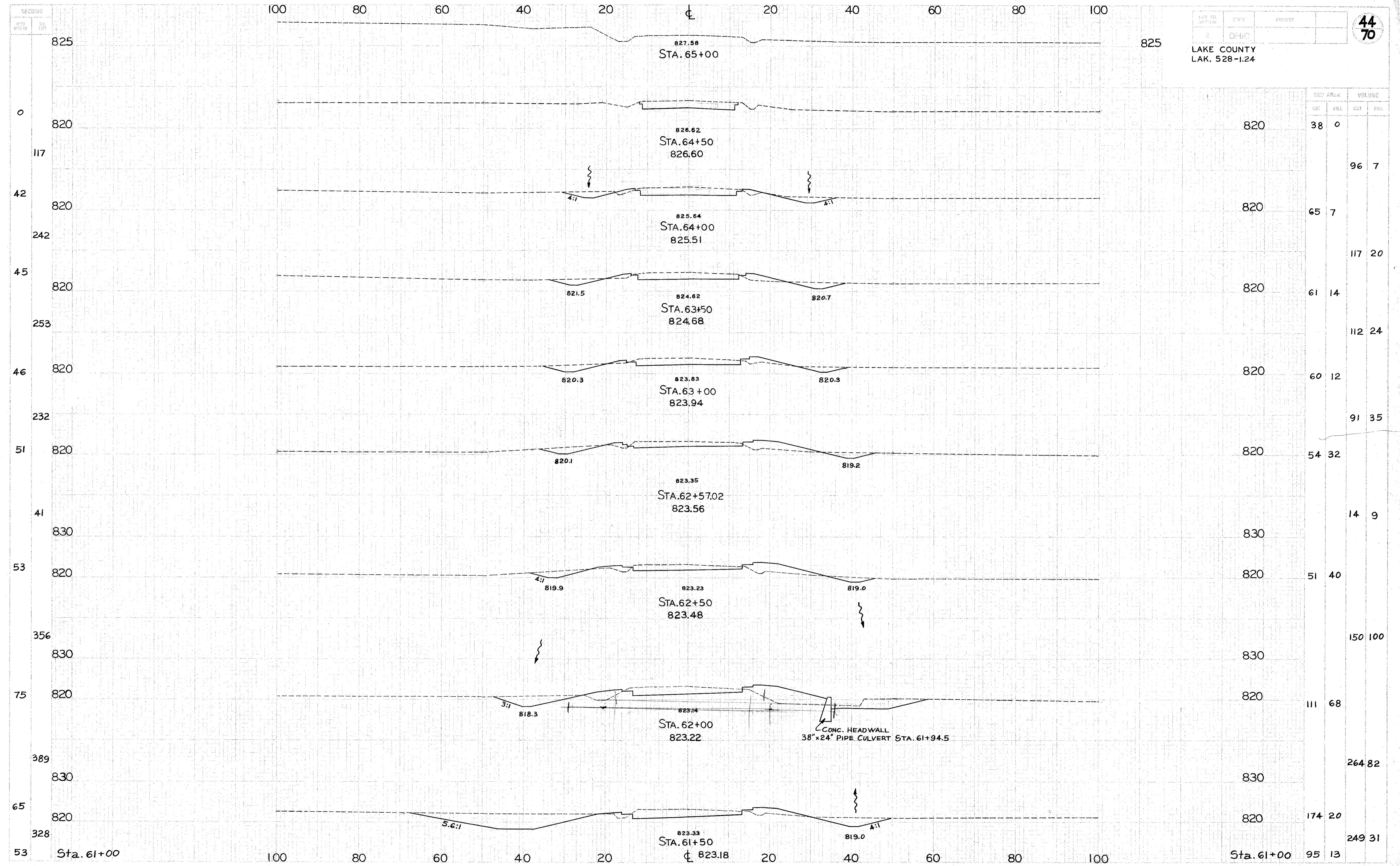
S.R. 528... CROSS SECTIONS... STA. 61+50 TO STA. 65+00
