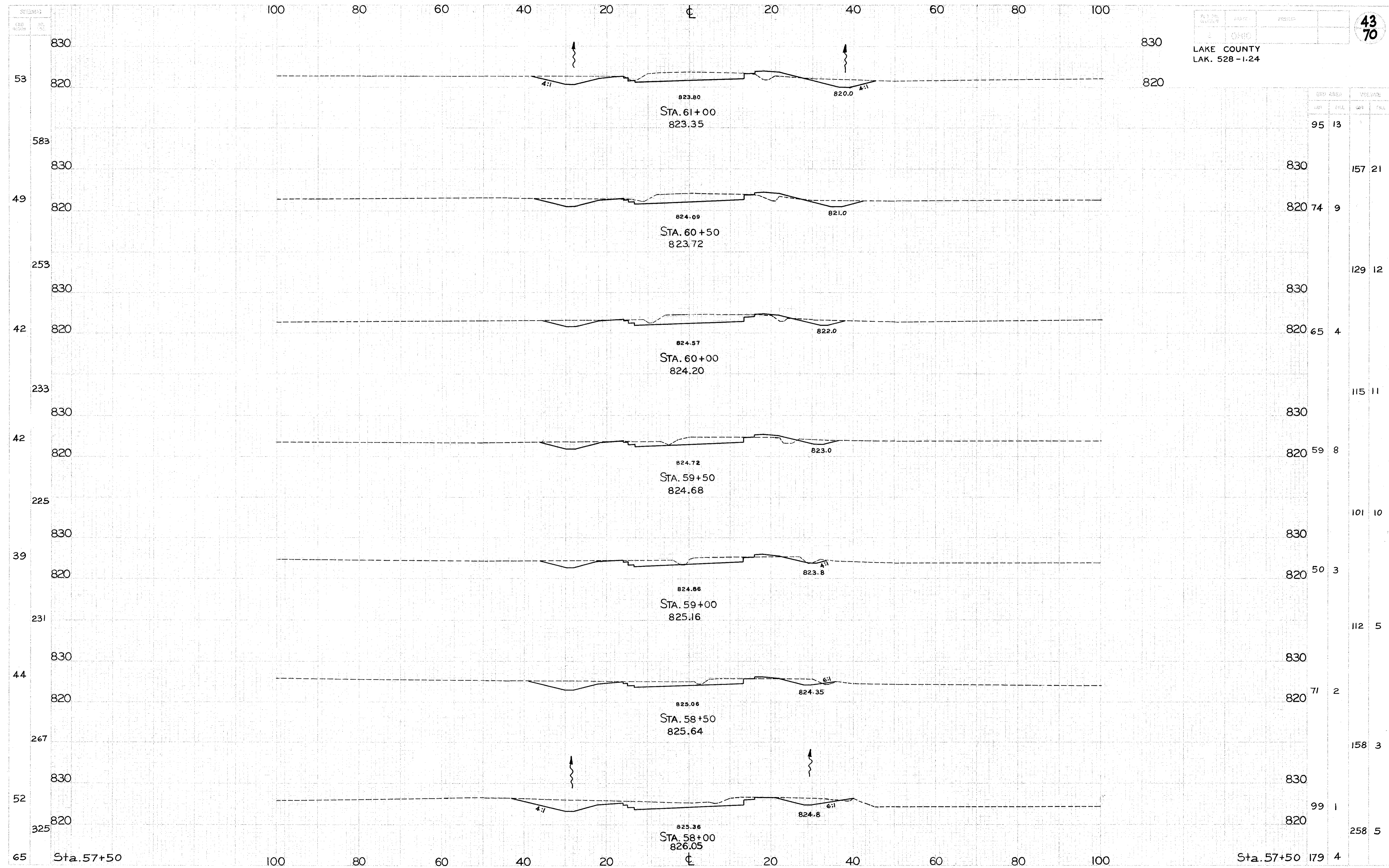
S.R. 528... CROSS SECTIONS... STA. 58+00 TO STA. 61+00
