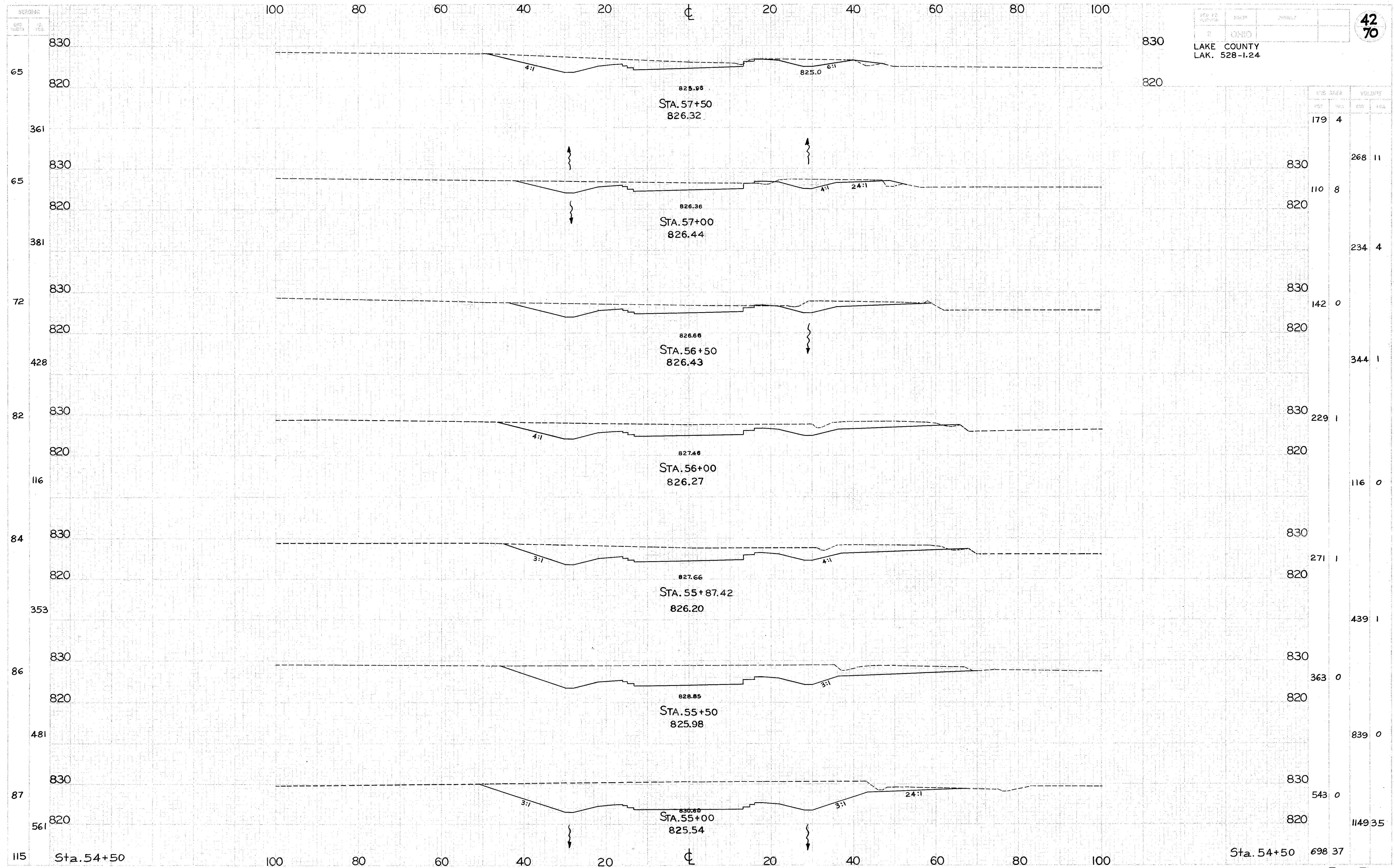
S.R. 528... CROSS SECTIONS... STA. 55+00 TO STA. 57+50
