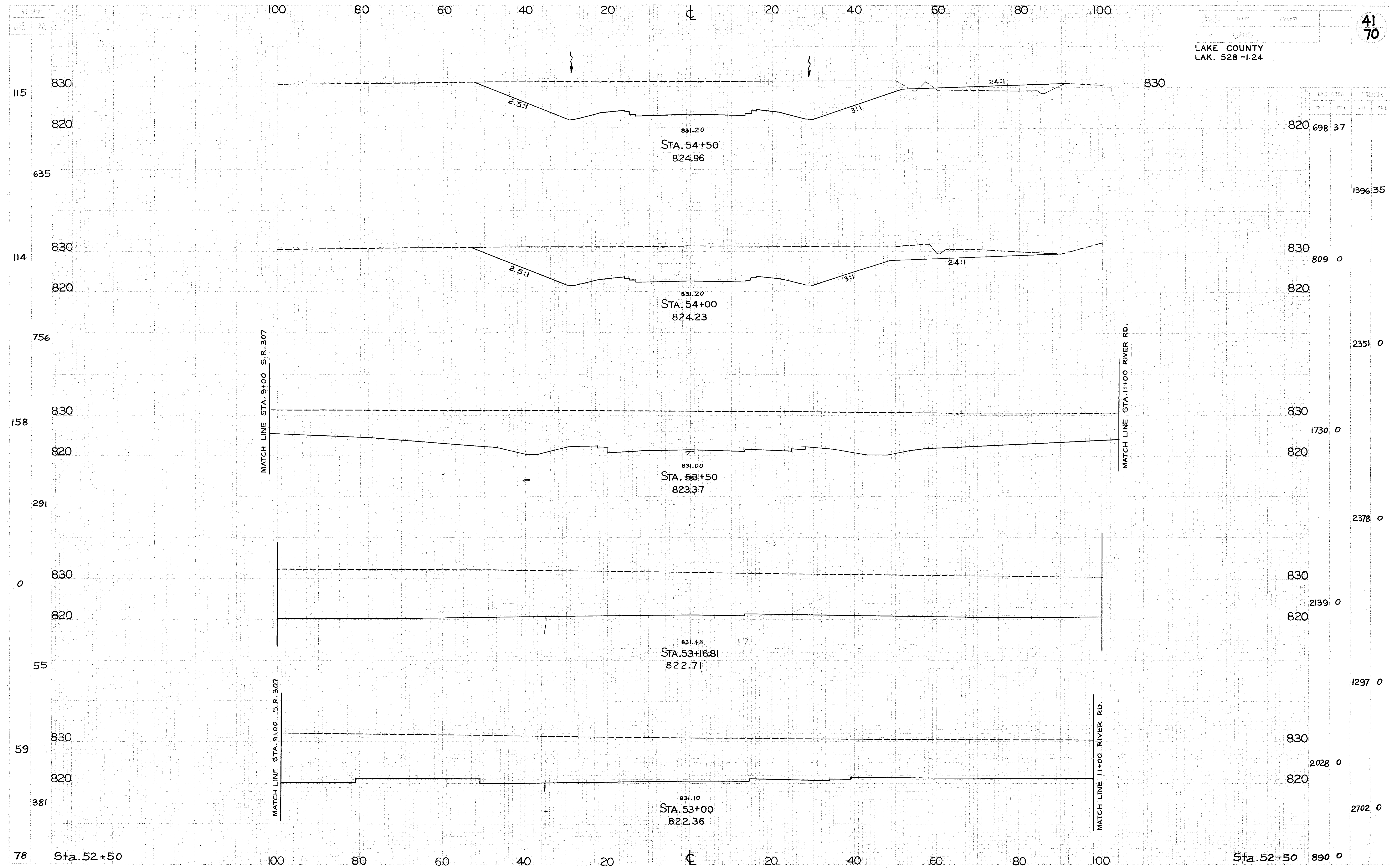
S.R. 528... CROSS SECTIONS ... STA. 53+00 TO STA. 54+50
