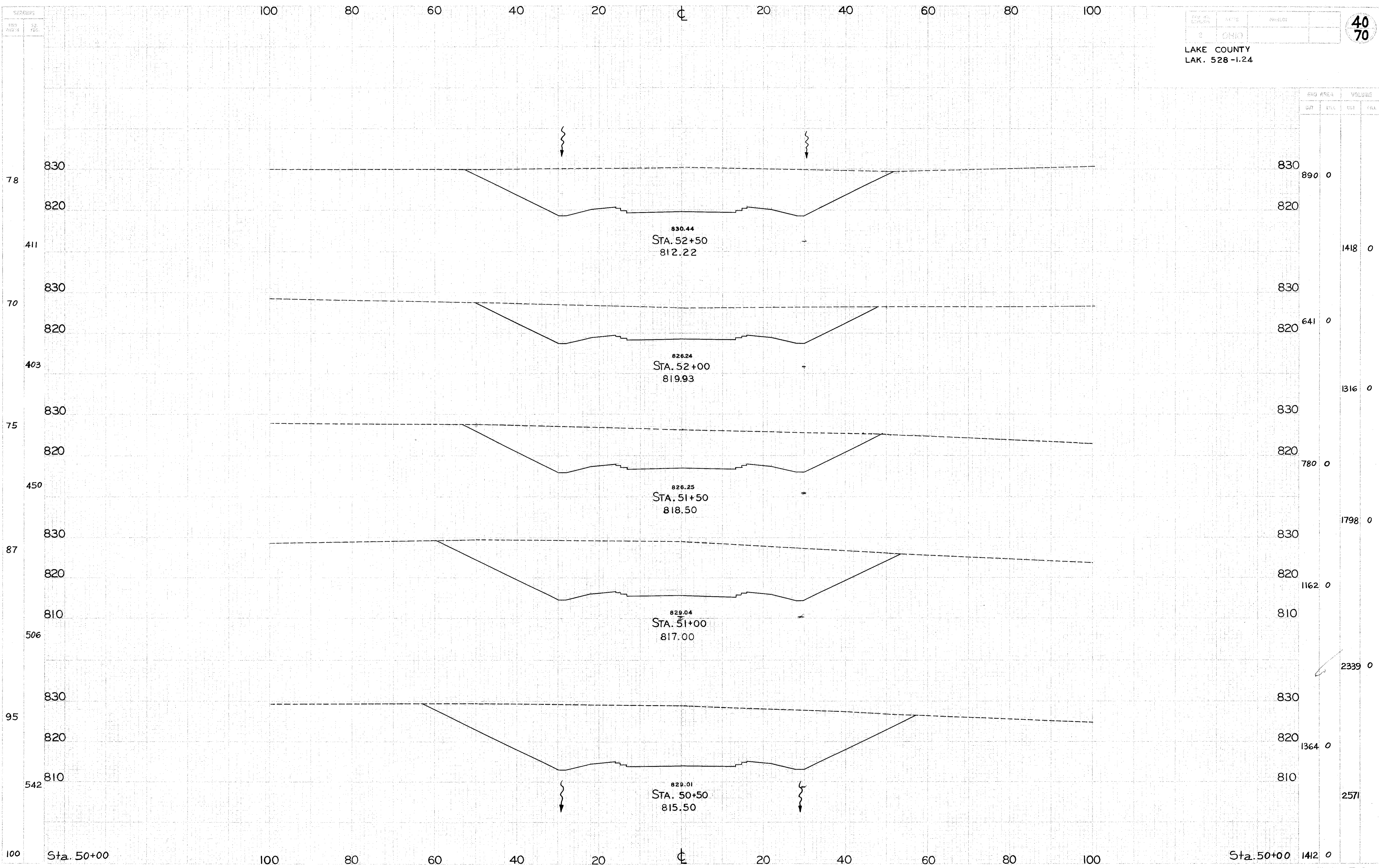
S.R. 528... CROSS SECTIONS... STA. 50+50 TO STA. 52+50
