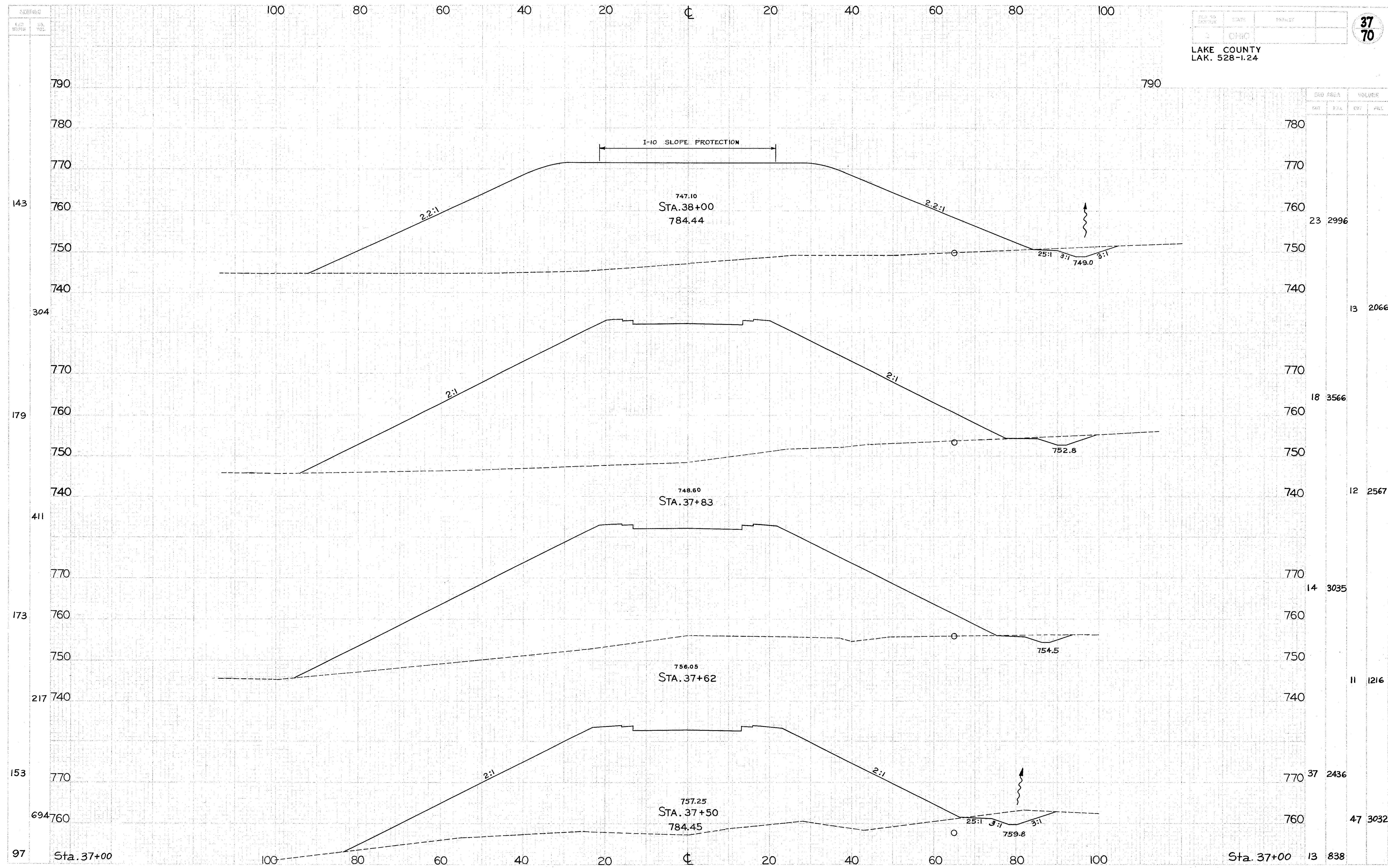
S.R. 528... CROSS SECTIONS ... STA. 37+50 TO STA. 38+00
