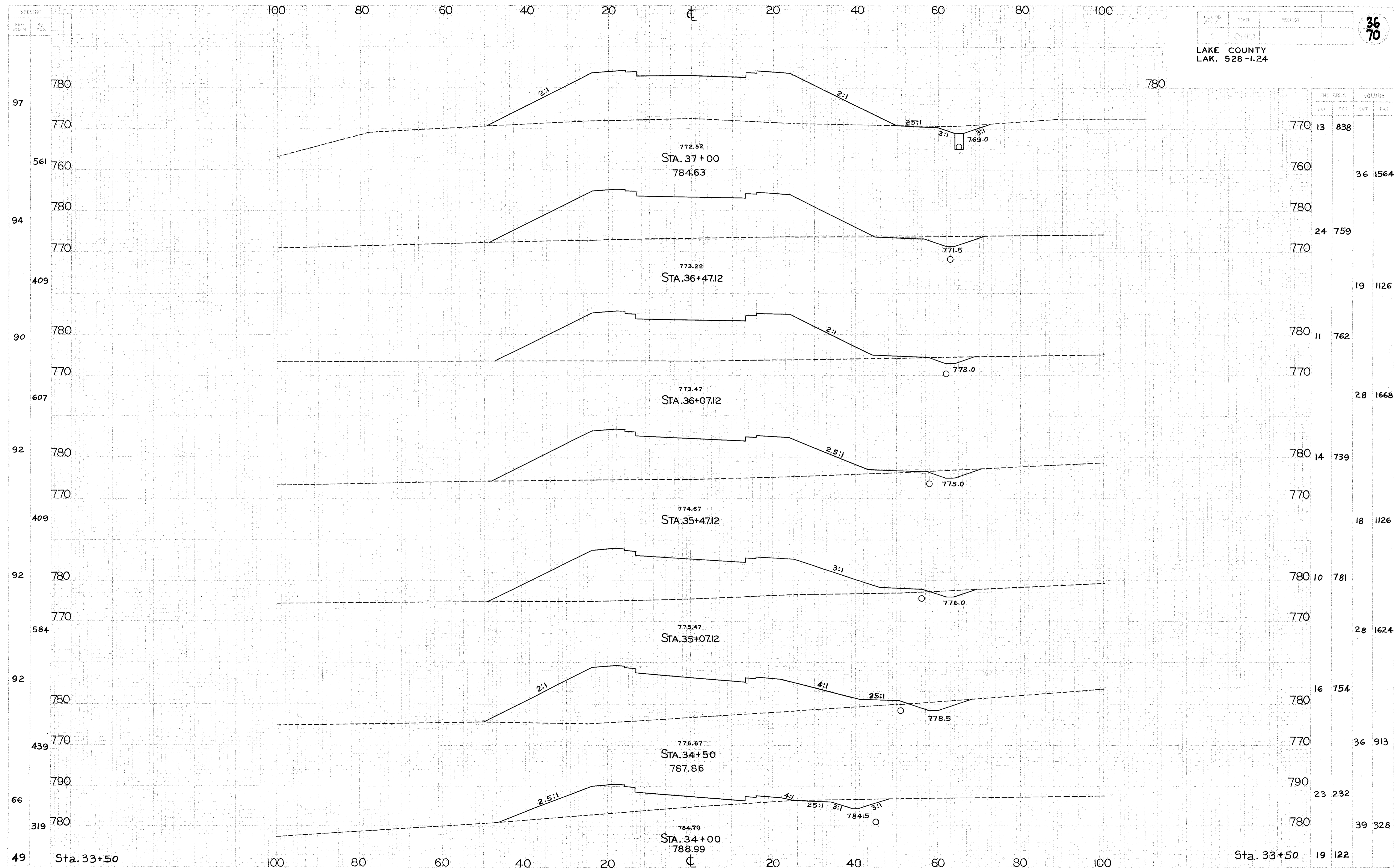
S.R. 528... CROSS SECTIONS... STA. 34+00 TO STA. 37+00
