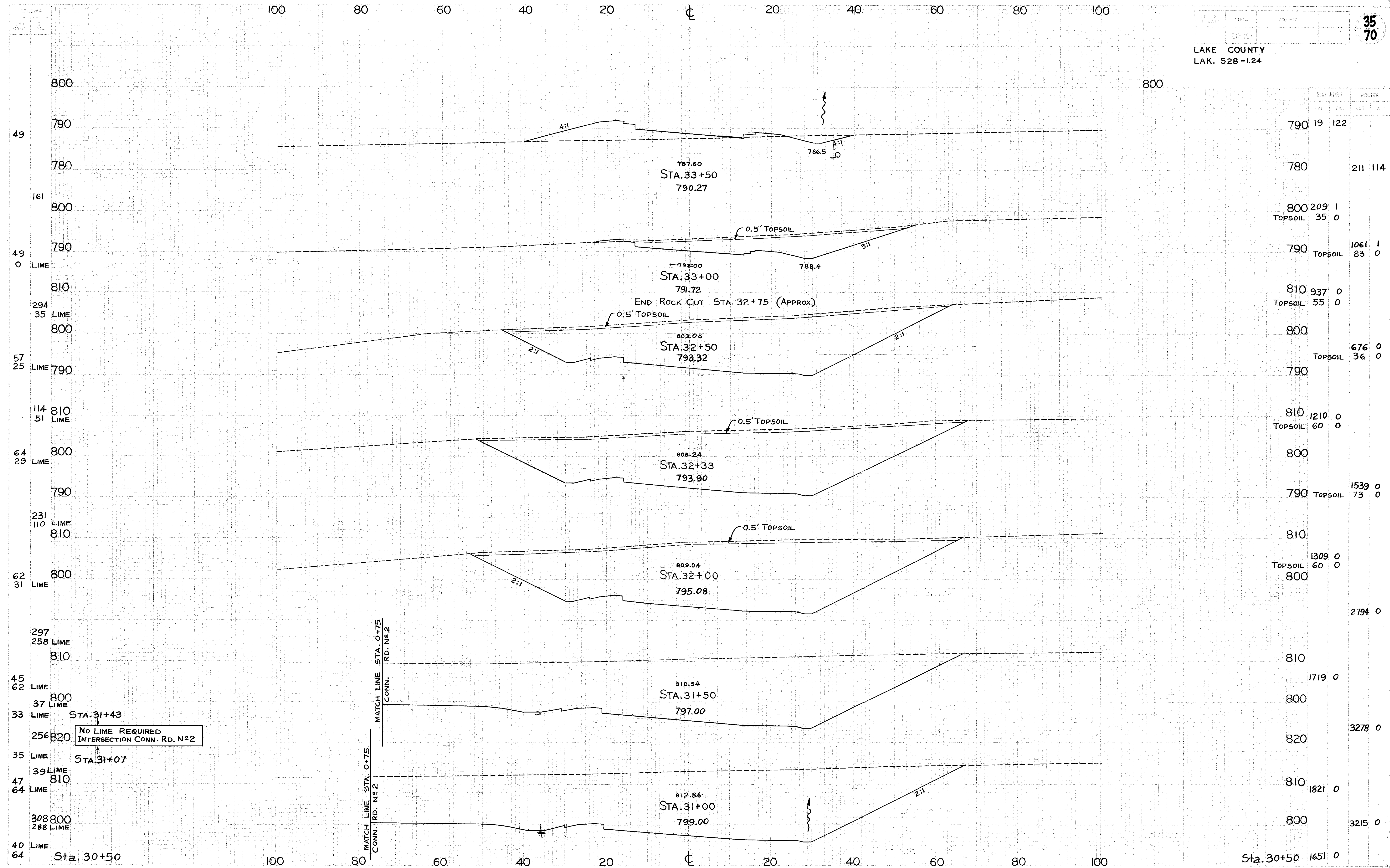
S.R. 528... CROSS SECTIONS... STA. 31+00 TO STA. 33+50
