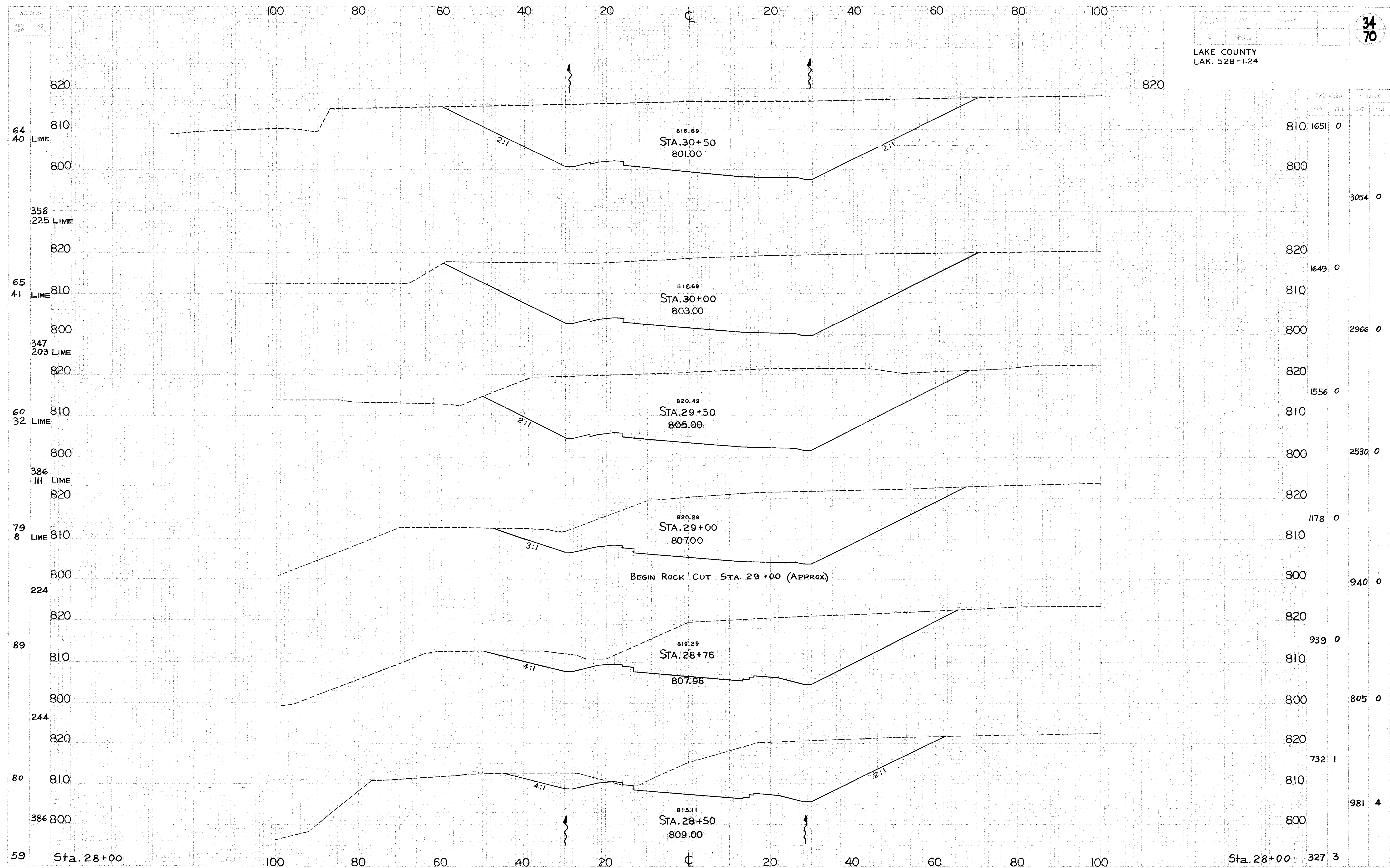
S.R. 528... CROSS SECTIONS... STA. 28+50 TO STA. 30+50
