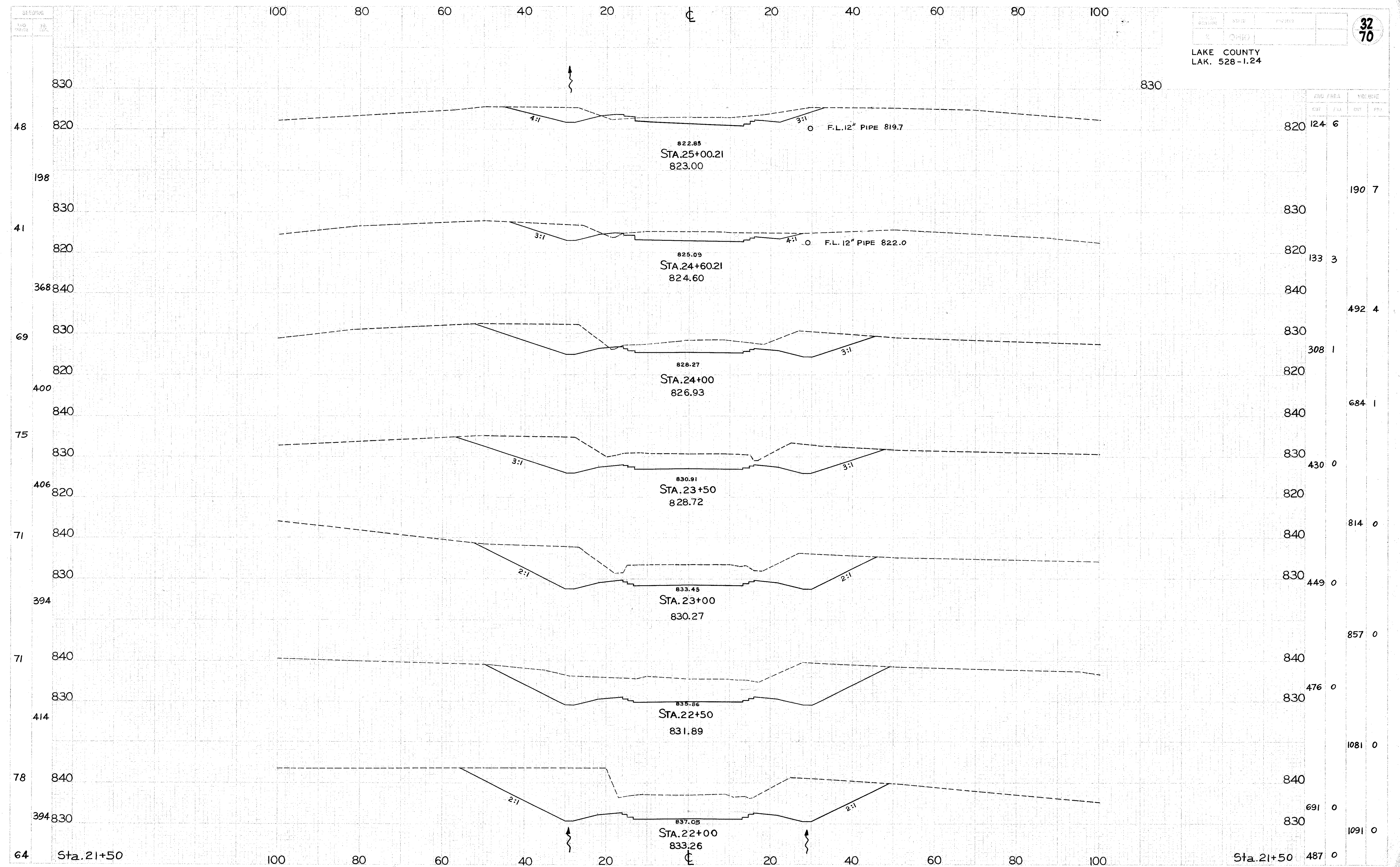
S.R. 528... CROSS SECTIONS... STA. 22+00 TO STA. 25+00.21
