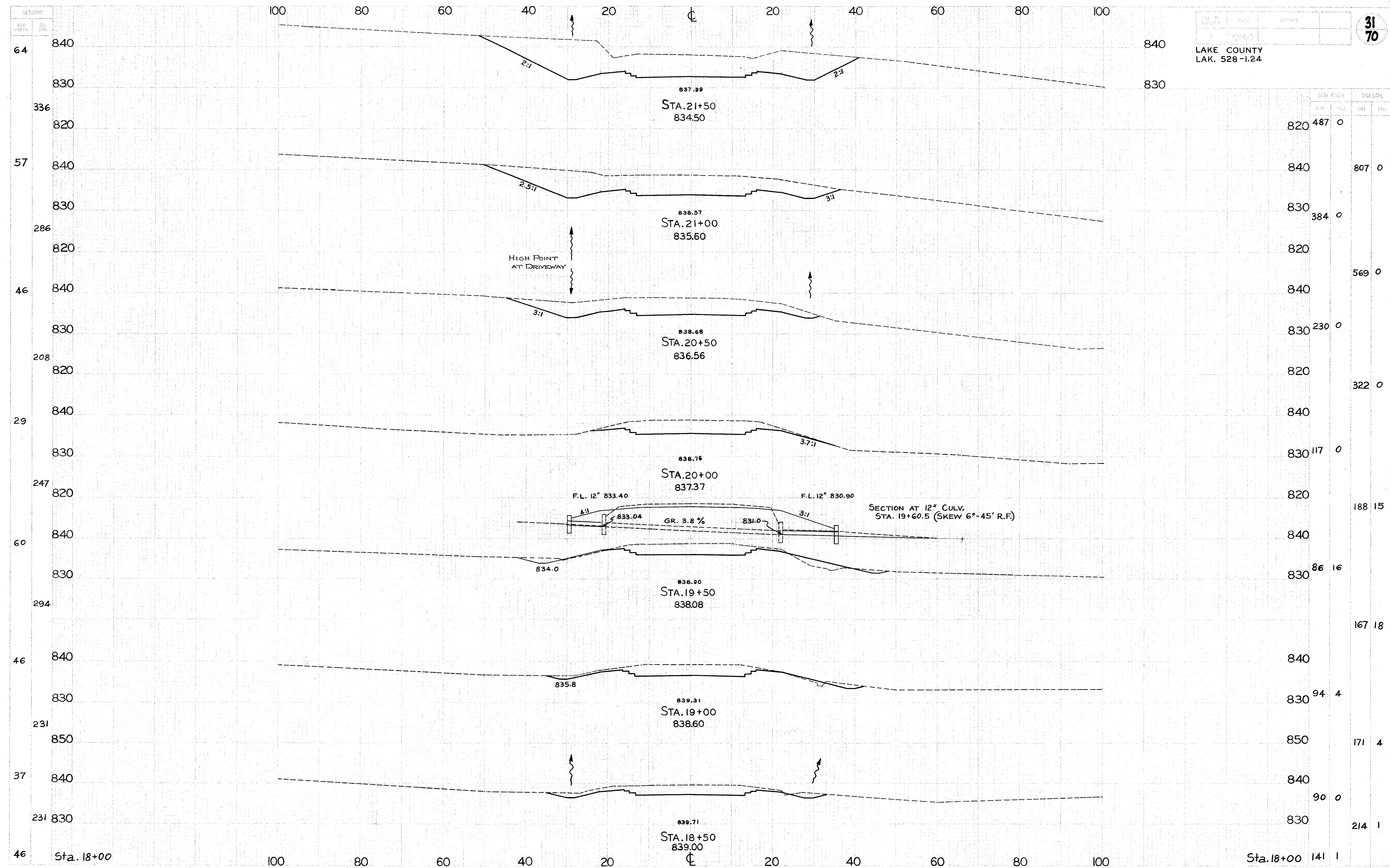
S.R. 528... CROSS SECTIONS... STA. 18+50 TO STA. 21+50
