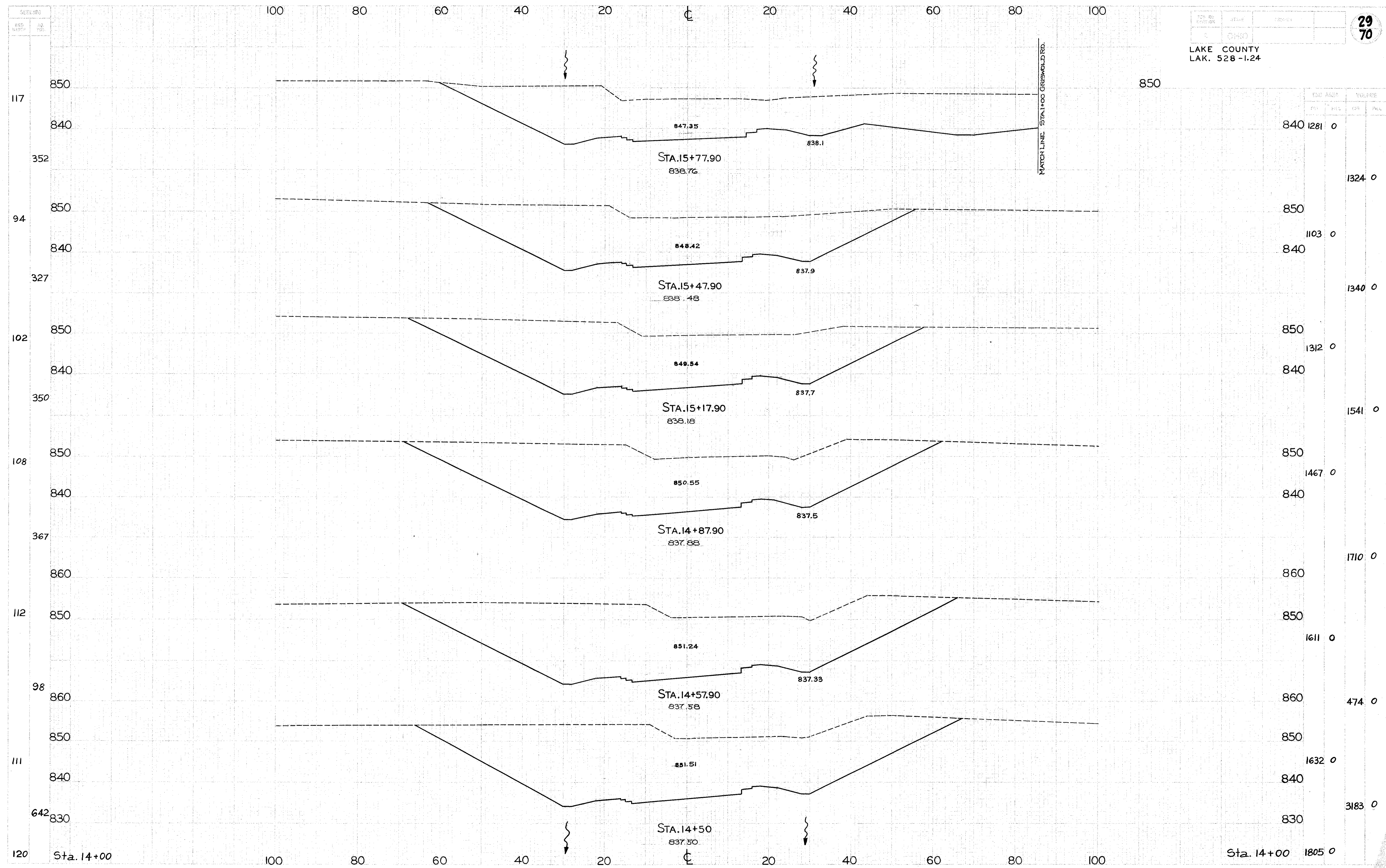
S.R. 528... CROSS SECTIONS... STA. 14+50 TO STA. 15+77.90
