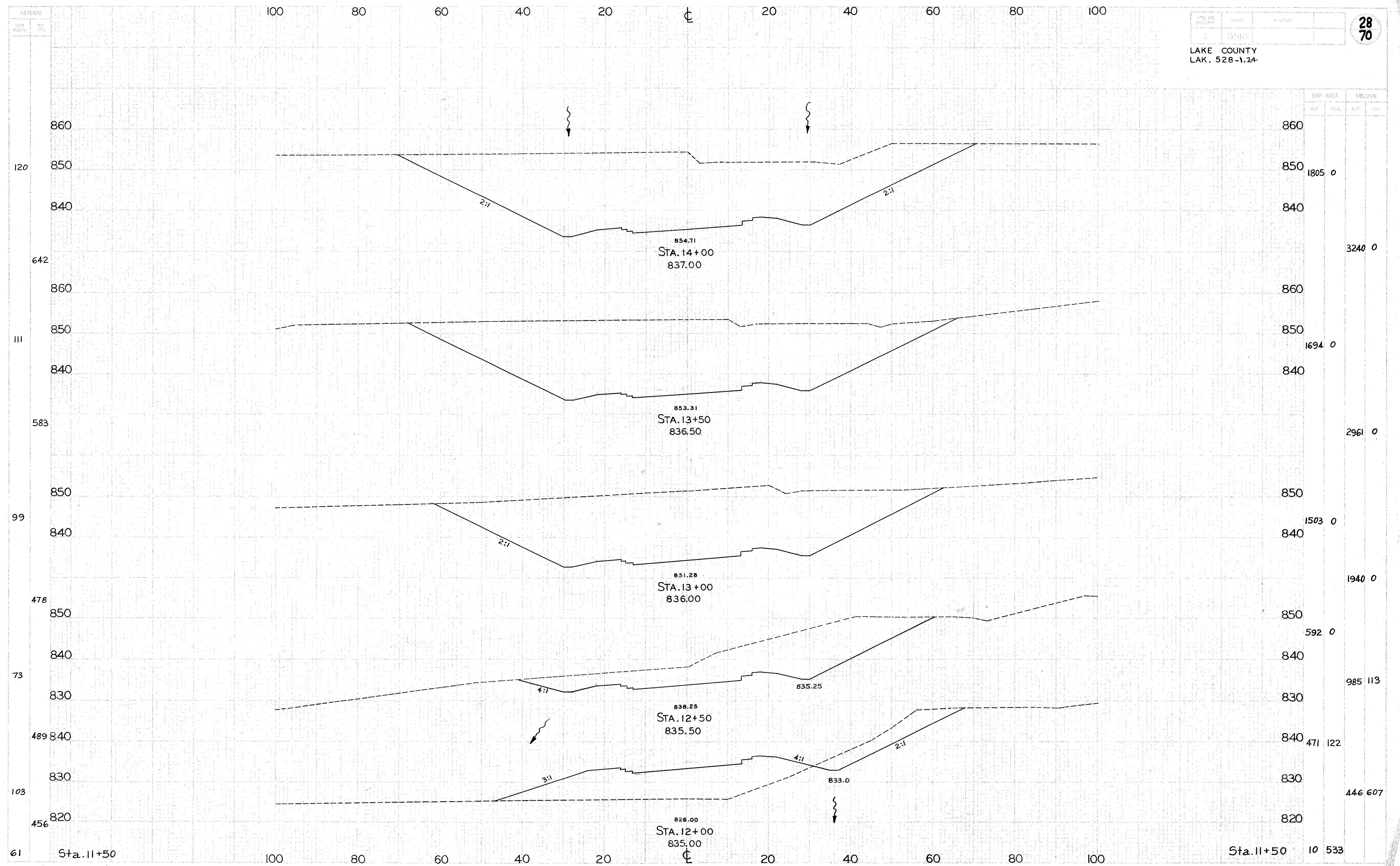
S.R. 528 ... CROSS SECTIONS ... STA. 12+00 TO STA. 14+00
